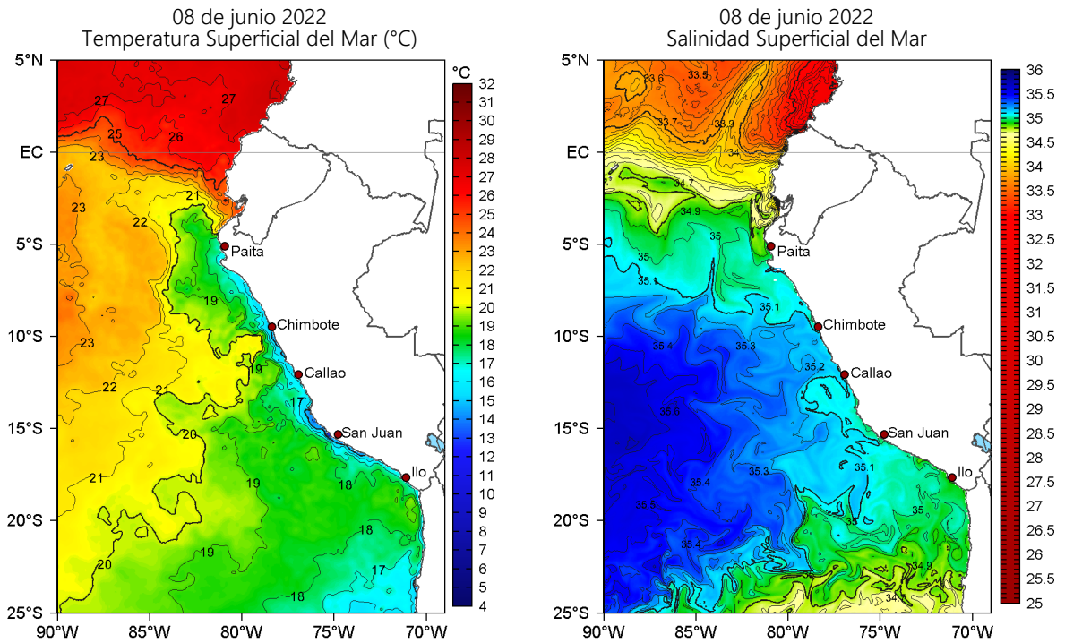
Figura 2. Temperatura superficial del mar (a la izquierda) y Salinidad superficial del mar (a la derecha) para el 08 de junio de 2022. Datos: OSTIA-UKMO-L4-GLOB-v2.0 (UK Met Office, 2012; Donlon et al, 2012) y Hybrid Coordinate Ocean Model v. GOFS 3.1 (HYCOM; Halliwell et al., 1998; 2000; Bleck, 2001), respectivamente.
