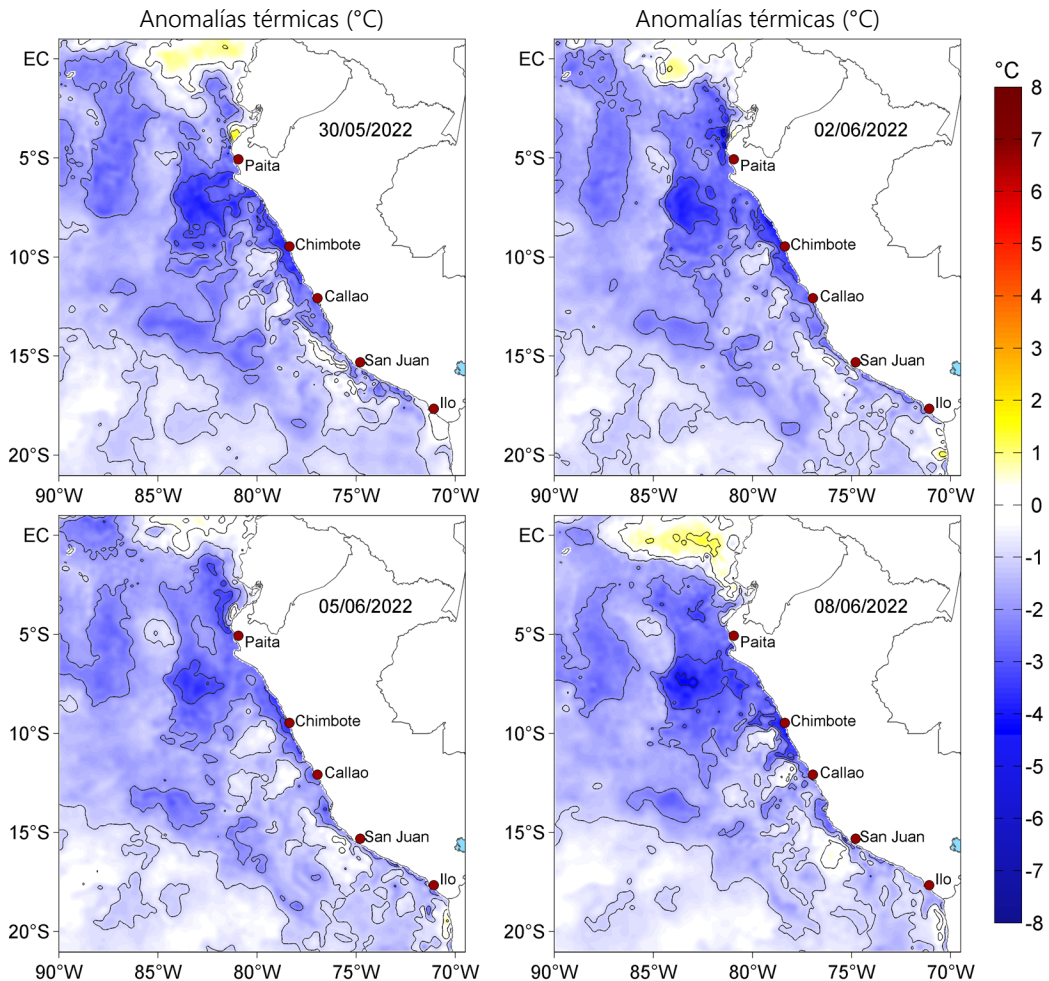
Figura 3. Anomalías de la temperatura superficial del mar (°C) para el 30 de mayo, así como para el 02, 05 y 08 de junio de 2022. Las anomalías se calcularon respecto de la climatología para el periodo 2007-2016. Datos: OSTIA-UKMO-L4-GLOB-v2.0 (UK Met Office, 2012; Donlon et al, 2012).
