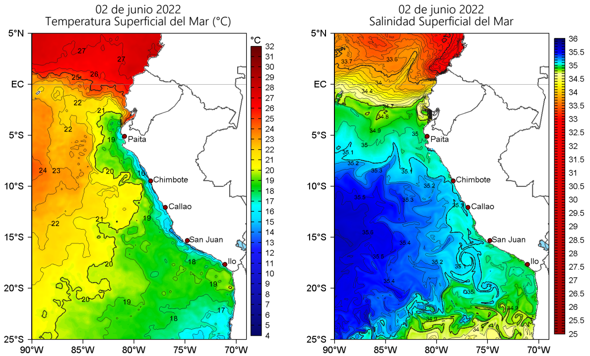
Figura 2. Temperatura superficial del mar (a la izquierda) y Salinidad superficial del mar (a la derecha) para el 02 de junio de 2022. Datos: OSTIA-UKMO-L4-GLOB-v2.0 (UK Met Office, 2012; Donlon et al, 2012) y Hybrid Coordinate Ocean Model v. GOFS 3.1 (HYCOM; Halliwell et al., 1998; 2000; Bleck, 2001), respectivamente.
