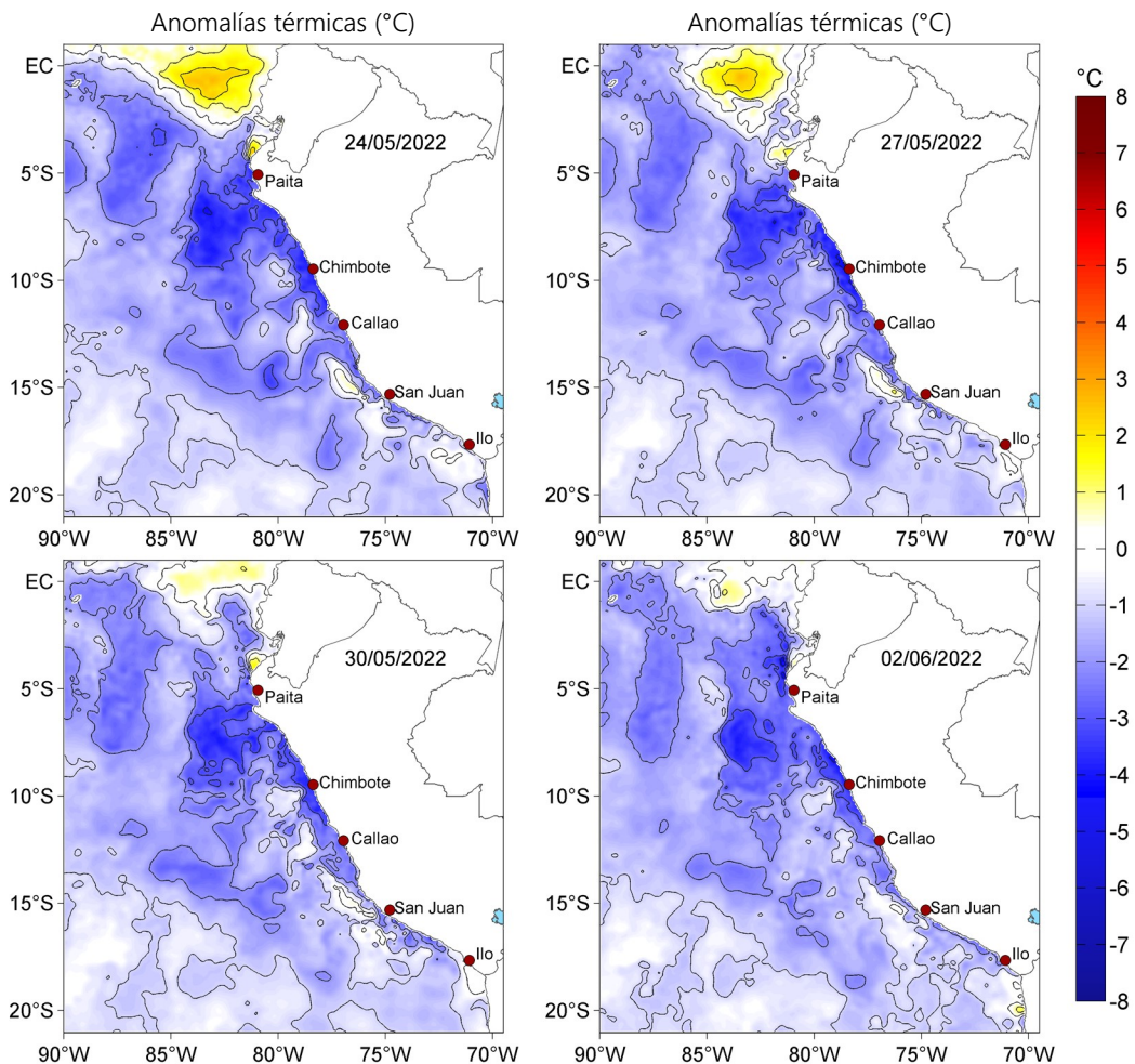
Figura 3. Anomalías de la temperatura superficial del mar (°C) para el 24, 27 y 30 de mayo, así como para el 02 de junio de 2022. Las anomalías se calcularon respecto de la climatología para el periodo 2007-2016. Datos: OSTIA-UKMO-L4-GLOB-v2.0 (UK Met Office, 2012; Donlon et al, 2012).
