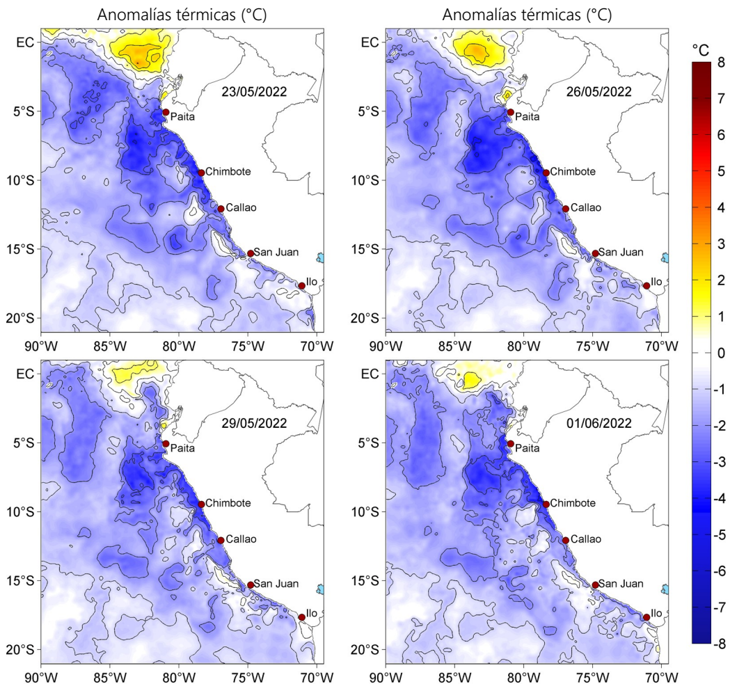
Figura 3. Anomalías de la temperatura superficial del mar (°C) para el 23, 26 y 29 de mayo, así como para el 01 de junio de 2022. Las anomalías se calcularon respecto de la climatología para el periodo 2007-2016. Datos: OSTIA-UKMO-L4-GLOB-v2.0 (UK Met Office, 2012; Donlon et al, 2012).
