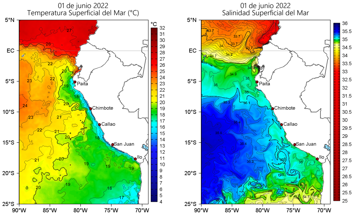
Figura 2. Temperatura superficial del mar (a la izquierda) y Salinidad superficial del mar (a la derecha) para el 01 de junio de 2022. Datos: OSTIA-UKMO-L4-GLOB-v2.0 (UK Met Office, 2012; Donlon et al, 2012) y Hybrid Coordinate Ocean Model v. GOFS 3.1 (HYCOM; Halliwell et al., 1998; 2000; Bleck, 2001), respectivamente.
