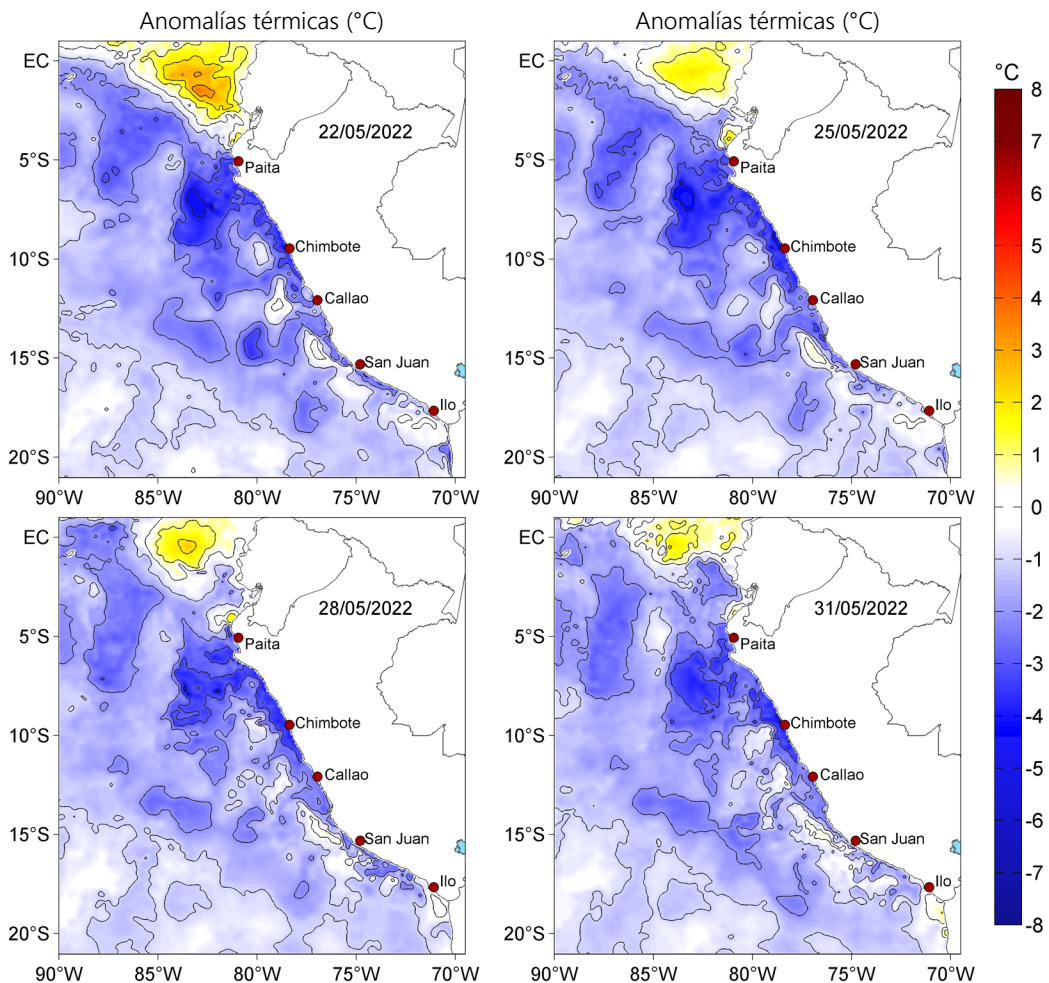
Figura 3. Anomalías de la temperatura superficial del mar (°C) para el 22, 25, 28 y 31 de mayo de 2022. Las anomalías se calcularon respecto de la climatología para el periodo 2007-2016. Datos: OSTIA-UKMO-L4-GLOB-v2.0 (UK Met Office, 2012; Donlon et al, 2012).
