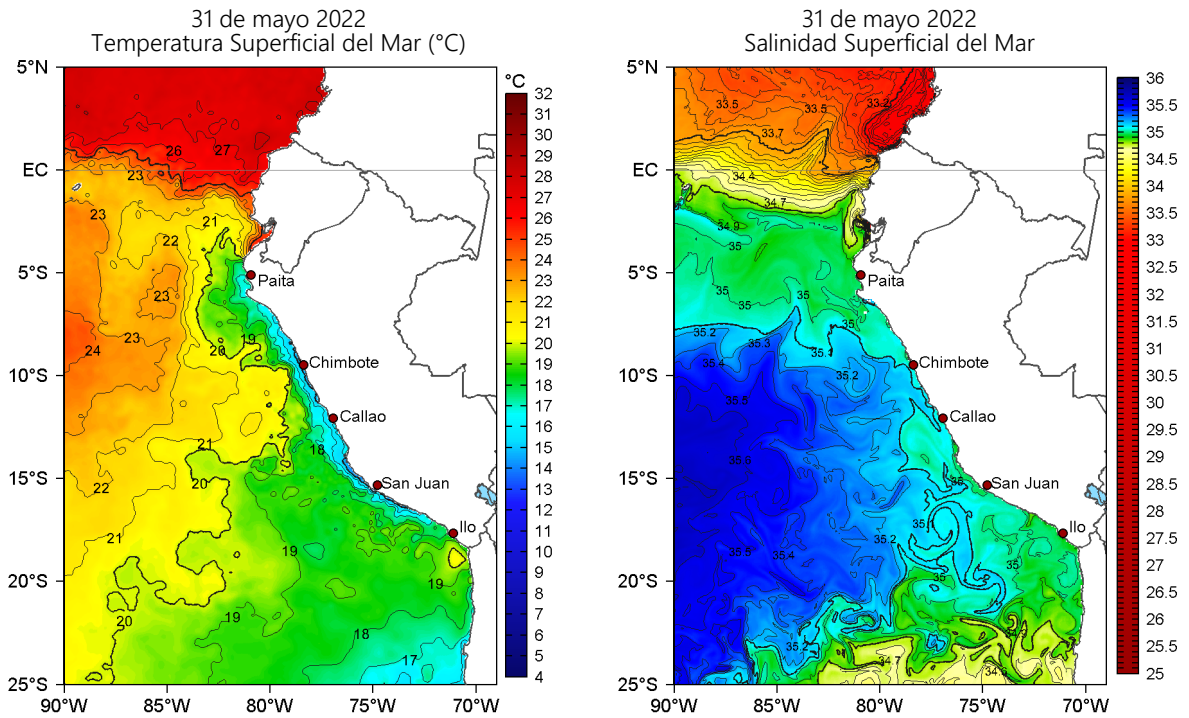
Figura 2. Temperatura superficial del mar (a la izquierda) y Salinidad superficial del mar (a la derecha) para el 31 de mayo de 2022. Datos: OSTIA-UKMO-L4-GLOB-v2.0 (UK Met Office, 2012; Donlon et al, 2012) y Hybrid Coordinate Ocean Model v. GOFS 3.1 (HYCOM; Halliwell et al., 1998; 2000; Bleck, 2001), respectivamente.
