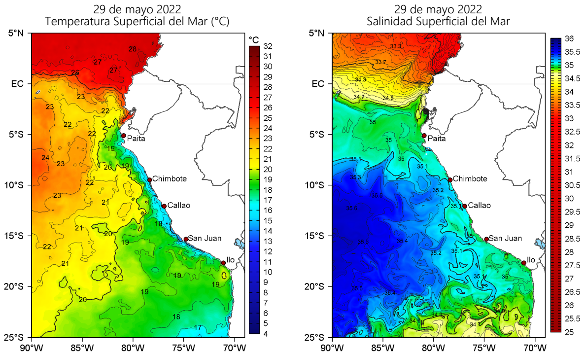
Figura 2. Temperatura superficial del mar (a la izquierda) y Salinidad superficial del mar (a la derecha) para el 29 de mayo de 2022. Datos: OSTIA-UKMO-L4-GLOB-v2.0 (UK Met Office, 2012; Donlon et al, 2012) y Hybrid Coordinate Ocean Model v. GOFS 3.1 (HYCOM; Halliwell et al., 1998; 2000; Bleck, 2001), respectivamente.
