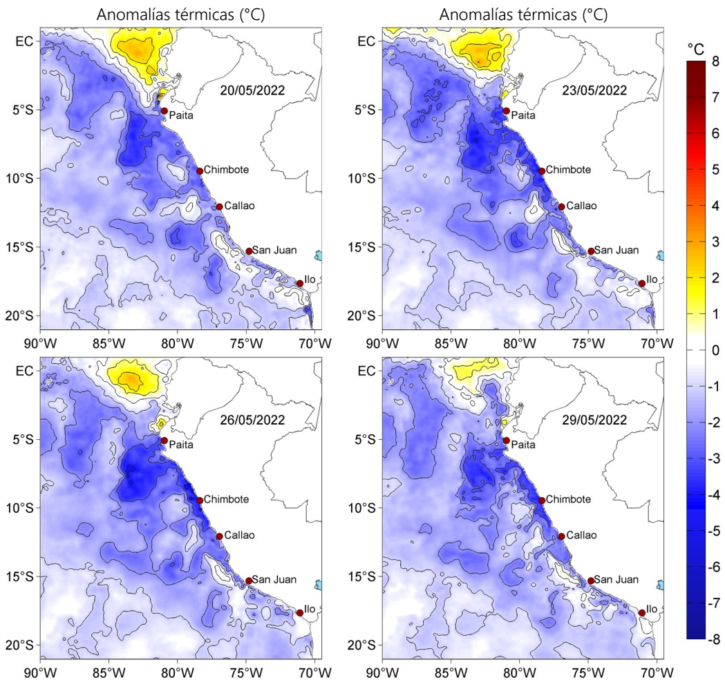
Figura 3. Anomalías de la temperatura superficial del mar (°C) para el 20, 23, 26 y 29 de mayo de 2022. Las anomalías se calcularon respecto de la climatología para el periodo 2007-2016. Datos: OSTIA-UKMO-L4-GLOB-v2.0 (UK Met Office, 2012; Donlon et al, 2012).
