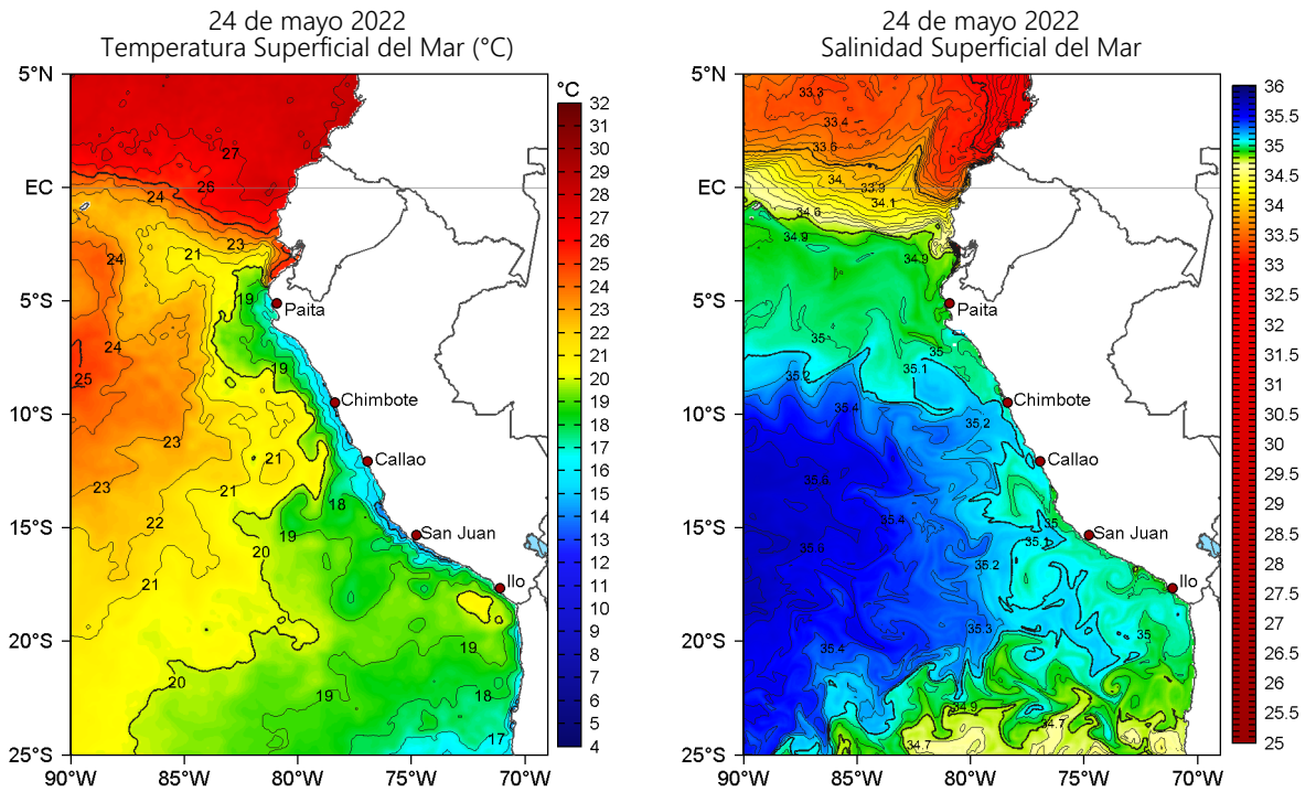
Figura 2. Temperatura superficial del mar (a la izquierda) y Salinidad superficial del mar (a la derecha) para el 24 de mayo de 2022. Datos: OSTIA-UKMO-L4-GLOB-v2.0 (UK Met Office, 2012; Donlon et al, 2012) y Hybrid Coordinate Ocean Model v. GOFS 3.1 (HYCOM; Halliwell et al., 1998; 2000; Bleck, 2001), respectivamente.
