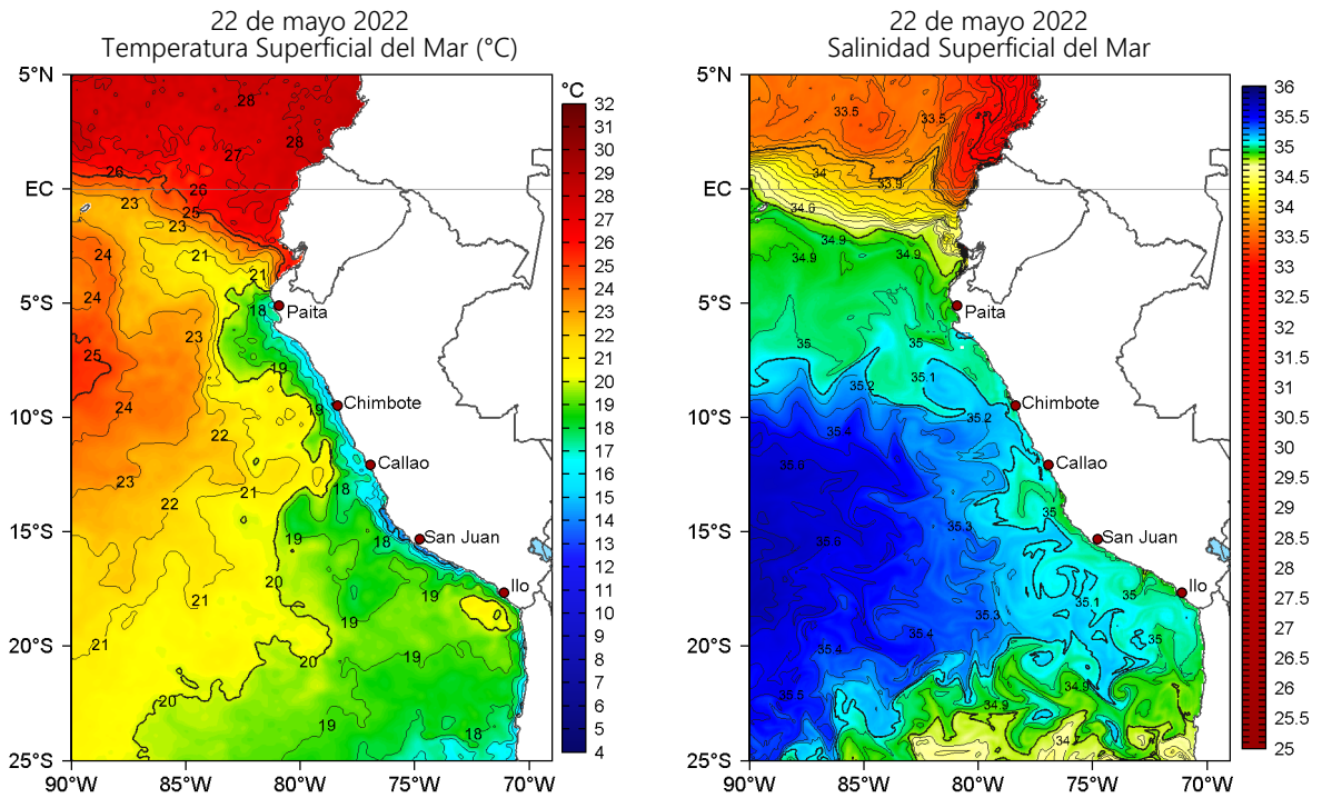
Figura 2. Temperatura superficial del mar (a la izquierda) y Salinidad superficial del mar (a la derecha) para el 22 de mayo de 2022. Datos: OSTIA-UKMO-L4-GLOB-v2.0 (UK Met Office, 2012; Donlon et al, 2012) y Hybrid Coordinate Ocean Model v. GOFS 3.1 (HYCOM; Halliwell et al., 1998; 2000; Bleck, 2001), respectivamente.
