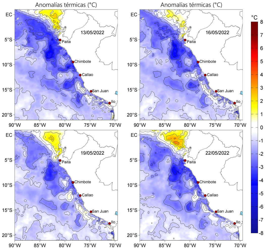
Figura 3. Anomalías de la temperatura superficial del mar (°C) para el 13, 16, 19 y 22 de mayo de 2022. Las anomalías se calcularon respecto de la climatología para el periodo 2007-2016. Datos: OSTIA-UKMO-L4-GLOB-v2.0 (UK Met Office, 2012; Donlon et al, 2012).
