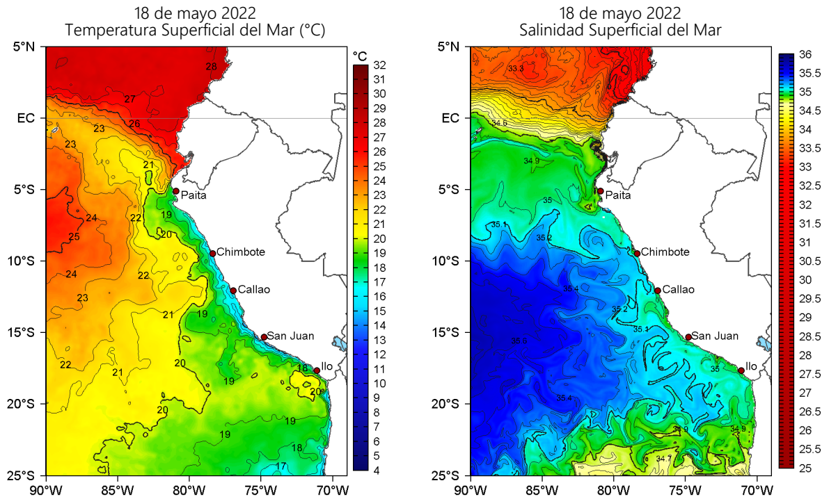
Figura 2. Temperatura superficial del mar (a la izquierda) y Salinidad superficial del mar (a la derecha) para el 18 de mayo de 2022. Datos: OSTIA-UKMO-L4-GLOB-v2.0 (UK Met Office, 2012; Donlon et al, 2012) y Hybrid Coordinate Ocean Model v. GOFS 3.1 (HYCOM; Halliwell et al., 1998; 2000; Bleck, 2001), respectivamente.
