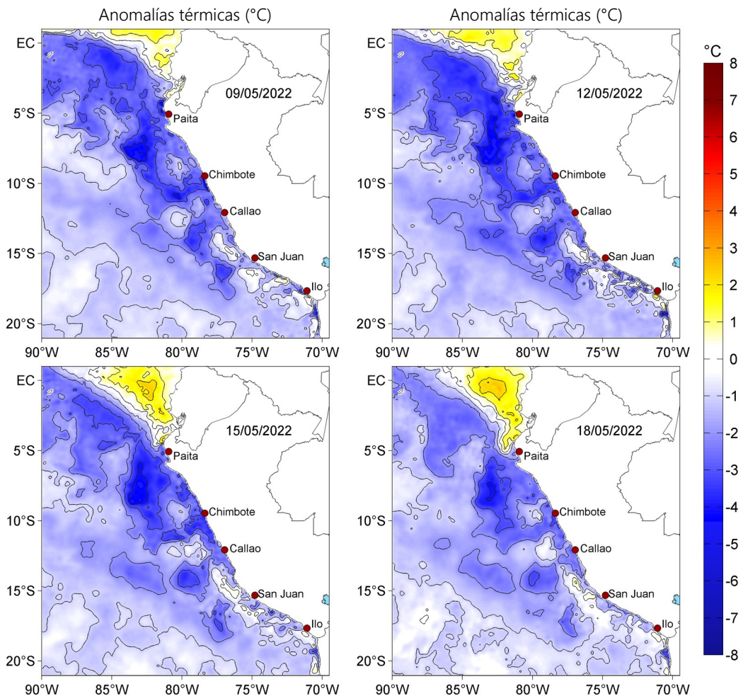
Figura 3. Anomalías de la temperatura superficial del mar (°C) para el 09, 12, 15 y 18 de mayo de 2022. Las anomalías se calcularon respecto de la climatología para el periodo 2007-2016. Datos: OSTIA-UKMO-L4-GLOB-v2.0 (UK Met Office, 2012; Donlon et al, 2012).
