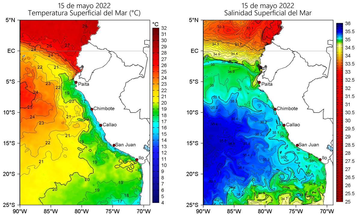
Figura 2. Temperatura superficial del mar (a la izquierda) y Salinidad superficial del mar (a la derecha) para el 15 de mayo de 2022. Datos: OSTIA-UKMO-L4-GLOB-v2.0 (UK Met Office, 2012; Donlon et al, 2012) y Hybrid Coordinate Ocean Model v. GOFS 3.1 (HYCOM; Halliwell et al., 1998; 2000; Bleck, 2001), respectivamente.
