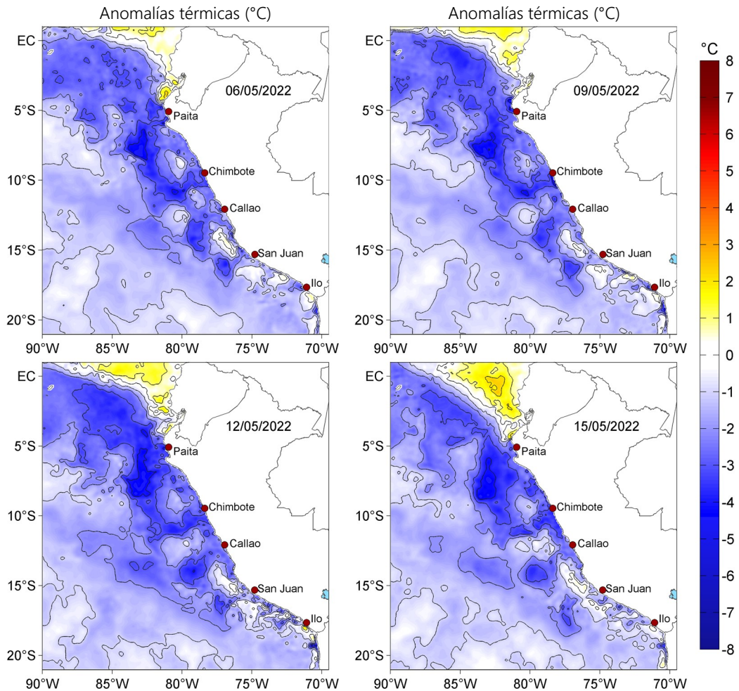
Figura 3. Anomalías de la temperatura superficial del mar (°C) para el 06, 09, 12 y 15 de mayo de 2022. Las anomalías se calcularon respecto de la climatología para el periodo 2007-2016. Datos: OSTIA-UKMO-L4-GLOB-v2.0 (UK Met Office, 2012; Donlon et al, 2012).
