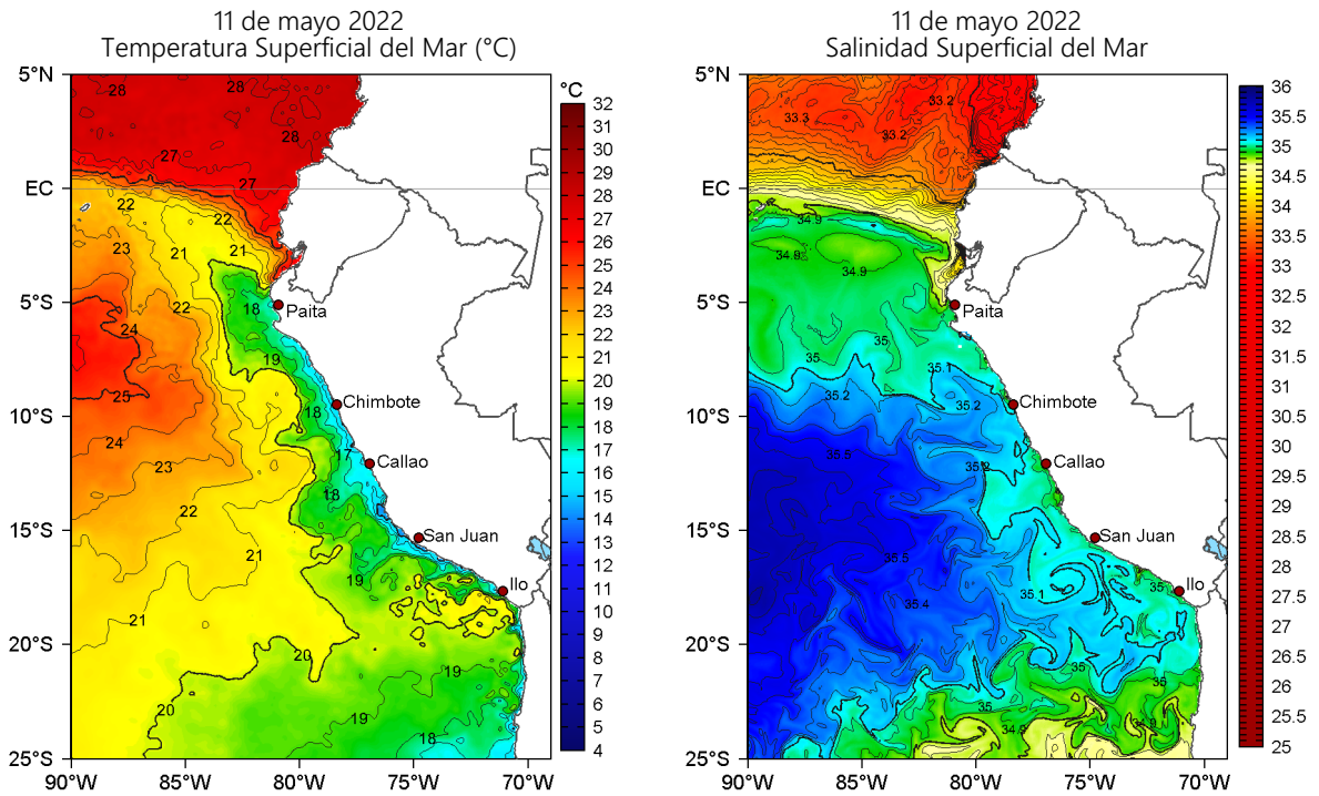
Figura 2. Temperatura superficial del mar (a la izquierda) y Salinidad superficial del mar (a la derecha) para el 11 de mayo de 2022. Datos: OSTIA-UKMO-L4-GLOB-v2.0 (UK Met Office, 2012; Donlon et al, 2012) y Hybrid Coordinate Ocean Model v. GOFS 3.1 (HYCOM; Halliwell et al., 1998; 2000; Bleck, 2001), respectivamente.
