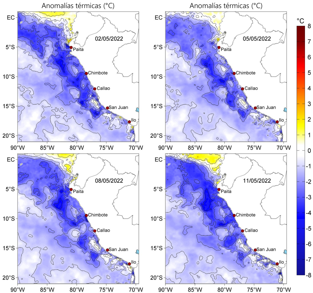
Figura 3. Anomalías de la temperatura superficial del mar (°C) para el 02, 05, 08 y 11 de mayo de 2022. Las anomalías se calcularon respecto de la climatología para el periodo 2007-2016. Datos: OSTIA-UKMO-L4-GLOB-v2.0 (UK Met Office, 2012; Donlon et al, 2012).
