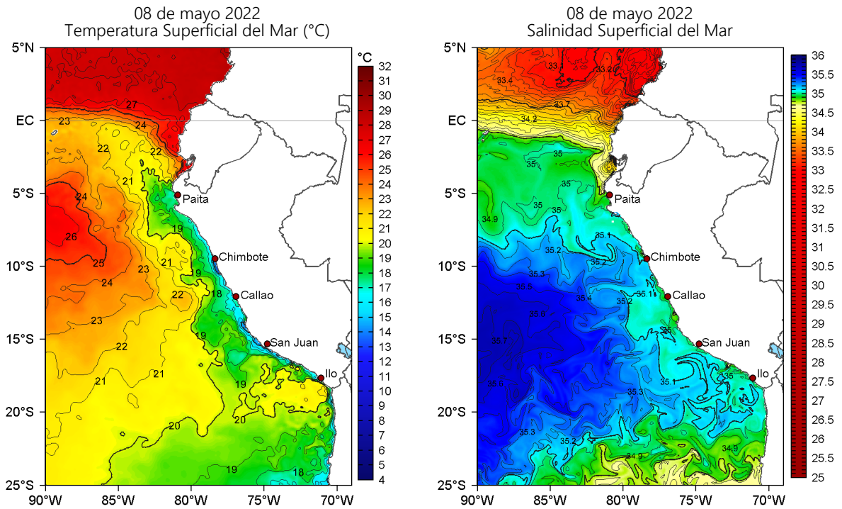
Figura 2. Temperatura superficial del mar (a la izquierda) y Salinidad superficial del mar (a la derecha) para el 08 de mayo de 2022. Datos: OSTIA-UKMO-L4-GLOB-v2.0 (UK Met Office, 2012; Donlon et al, 2012) y Hybrid Coordinate Ocean Model v. GOFS 3.1 (HYCOM; Halliwell et al., 1998; 2000; Bleck, 2001), respectivamente.
