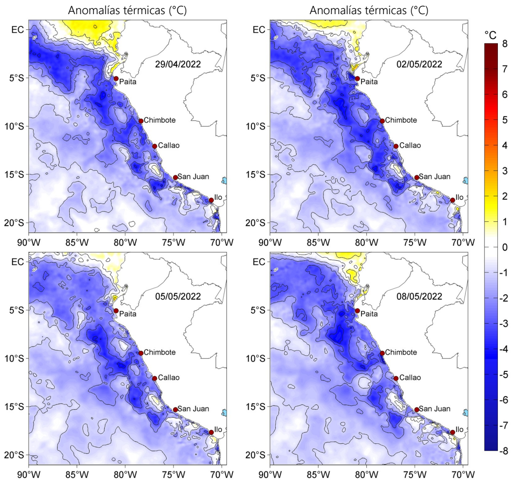
Figura 3. Anomalías de la temperatura superficial del mar (°C) para el 29 de abril, así como para el 02, 05 y 08 de mayo de 2022. Las anomalías se calcularon respecto de la climatología para el periodo 2007-2016. Datos: OSTIA-UKMO-L4-GLOB-v2.0 (UK Met Office, 2012; Donlon et al, 2012).
