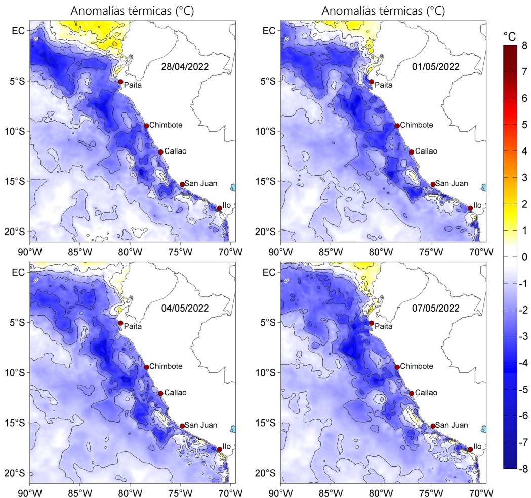
Figura 3. Anomalías de la temperatura superficial del mar (°C) para el 28 de abril, así como para el 01, 04 y 07 de mayo de 2022. Las anomalías se calcularon respecto de la climatología para el periodo 2007-2016. Datos: OSTIA-UKMO-L4-GLOB-v2.0 (UK Met Office, 2012; Donlon et al, 2012).
