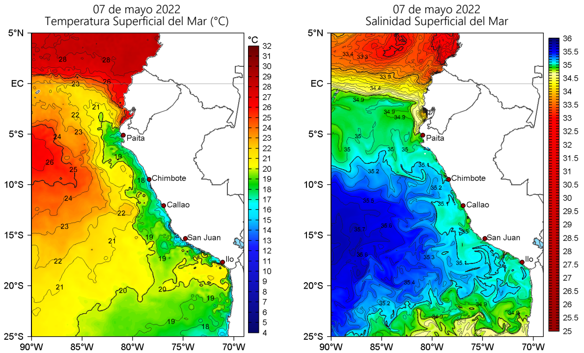
Figura 2. Temperatura superficial del mar (a la izquierda) y Salinidad superficial del mar (a la derecha) para el 07 de mayo de 2022. Datos: OSTIA-UKMO-L4-GLOB-v2.0 (UK Met Office, 2012; Donlon et al, 2012) y Hybrid Coordinate Ocean Model v. GOFS 3.1 (HYCOM; Halliwell et al., 1998; 2000; Bleck, 2001), respectivamente.
