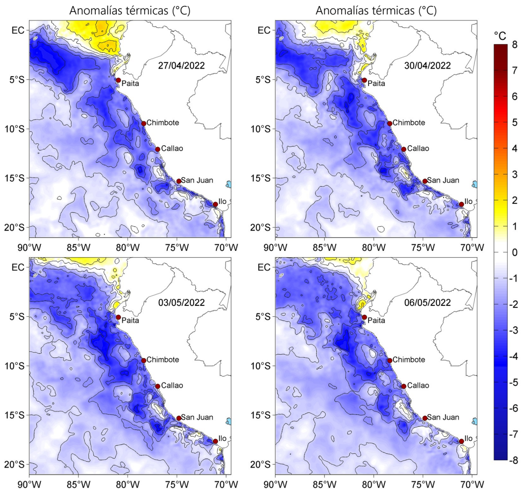
Figura 3. Anomalías de la temperatura superficial del mar (°C) para el 27 y 30 de abril, así como para el 03 y 06 de mayo de 2022. Las anomalías se calcularon respecto de la climatología para el periodo 2007-2016. Datos: OSTIA-UKMO-L4-GLOB-v2.0 (UK Met Office, 2012; Donlon et al, 2012).
