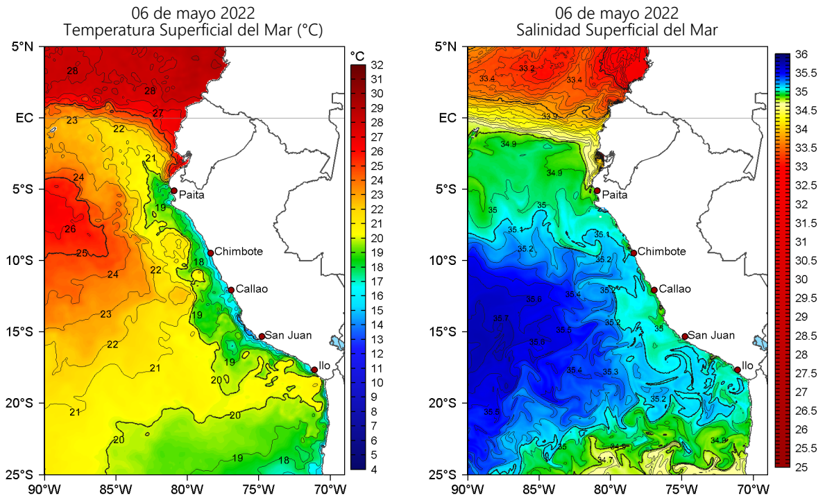
Figura 2. Temperatura superficial del mar (a la izquierda) y Salinidad superficial del mar (a la derecha) para el 06 de mayo de 2022. Datos: OSTIA-UKMO-L4-GLOB-v2.0 (UK Met Office, 2012; Donlon et al, 2012) y Hybrid Coordinate Ocean Model v. GOFS 3.1 (HYCOM; Halliwell et al., 1998; 2000; Bleck, 2001), respectivamente.
