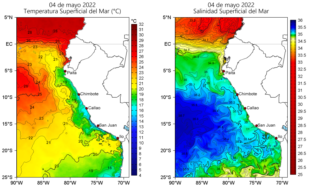
Figura 2. Temperatura superficial del mar (a la izquierda) y Salinidad superficial del mar (a la derecha) para el 04 de mayo de 2022. Datos: OSTIA-UKMO-L4-GLOB-v2.0 (UK Met Office, 2012; Donlon et al, 2012) y Hybrid Coordinate Ocean Model v. GOFS 3.1 (HYCOM; Halliwell et al., 1998; 2000; Bleck, 2001), respectivamente.
