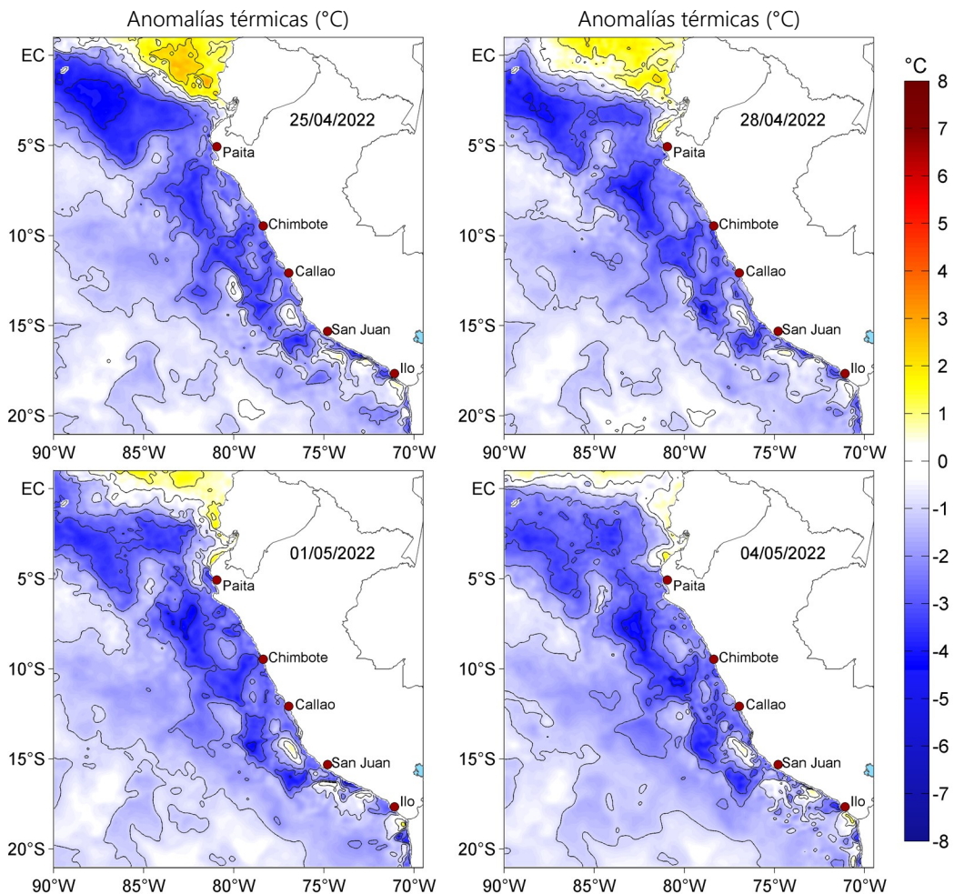
Figura 3. Anomalías de la temperatura superficial del mar (°C) para el 25 y 28 de abril, así como para el 01 y 04 de mayo de 2022. Las anomalías se calcularon respecto de la climatología para el periodo 2007-2016. Datos: OSTIA-UKMO-L4-GLOB-v2.0 (UK Met Office, 2012; Donlon et al, 2012).
