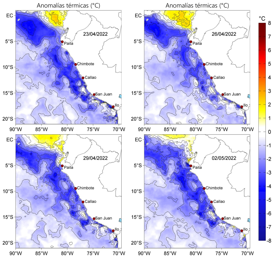
Figura 3. Anomalías de la temperatura superficial del mar (°C) para el 23, 26 y 29 de abril, así como para el 02 de mayo de 2022. Las anomalías se calcularon respecto de la climatología para el periodo 2007-2016. Datos: OSTIA-UKMO-L4-GLOB-v2.0 (UK Met Office, 2012; Donlon et al, 2012).
