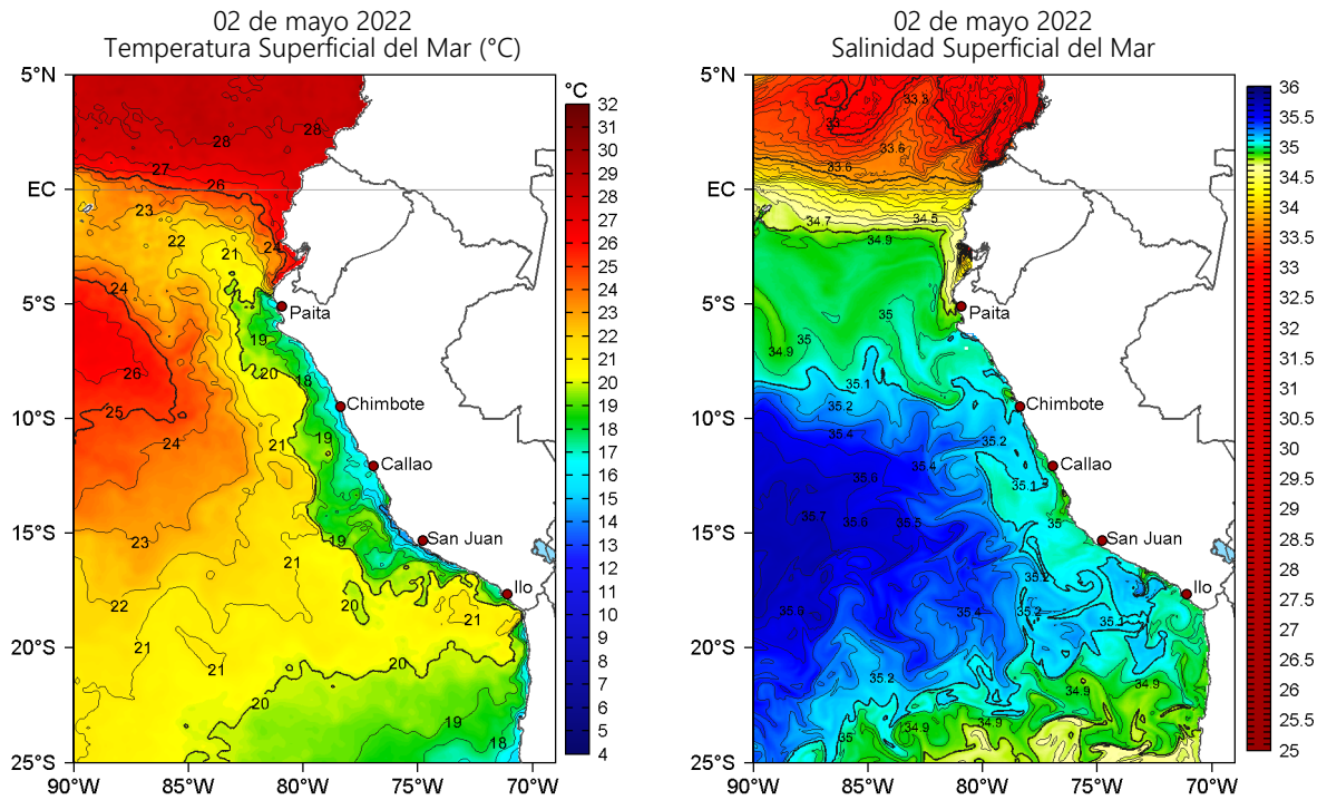
Figura 2. Temperatura superficial del mar (a la izquierda) y Salinidad superficial del mar (a la derecha) para el 02 de mayo de 2022. Datos: OSTIA-UKMO-L4-GLOB-v2.0 (UK Met Office, 2012; Donlon et al, 2012) y Hybrid Coordinate Ocean Model v. GOFS 3.1 (HYCOM; Halliwell et al., 1998; 2000; Bleck, 2001), respectivamente.
