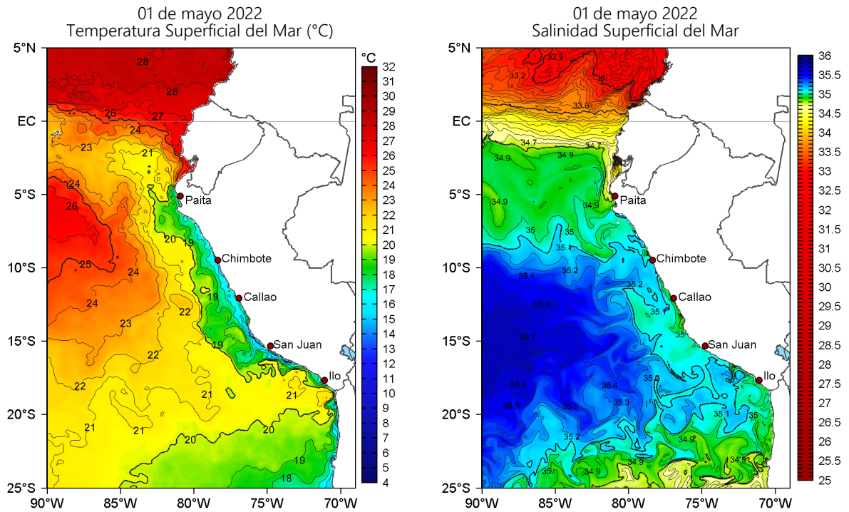
Figura 2. Temperatura superficial del mar (a la izquierda) y Salinidad superficial del mar (a la derecha) para el 01 de mayo de 2022. Datos: OSTIA-UKMO-L4-GLOB-v2.0 (UK Met Office, 2012; Donlon et al, 2012) y Hybrid Coordinate Ocean Model v. GOFS 3.1 (HYCOM; Halliwell et al., 1998; 2000; Bleck, 2001), respectivamente.
