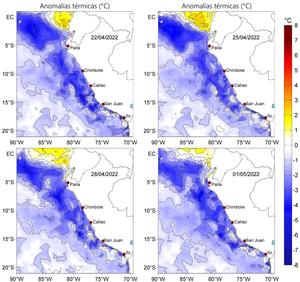
Figura 3. Anomalías de la temperatura superficial del mar (°C) para el 22, 25 y 28 de abril, así como para el 01 de mayo de 2022. Las anomalías se calcularon respecto de la climatología para el periodo 2007-2016. Datos: OSTIA-UKMO-L4-GLOB-v2.0 (UK Met Office, 2012; Donlon et al, 2012).
