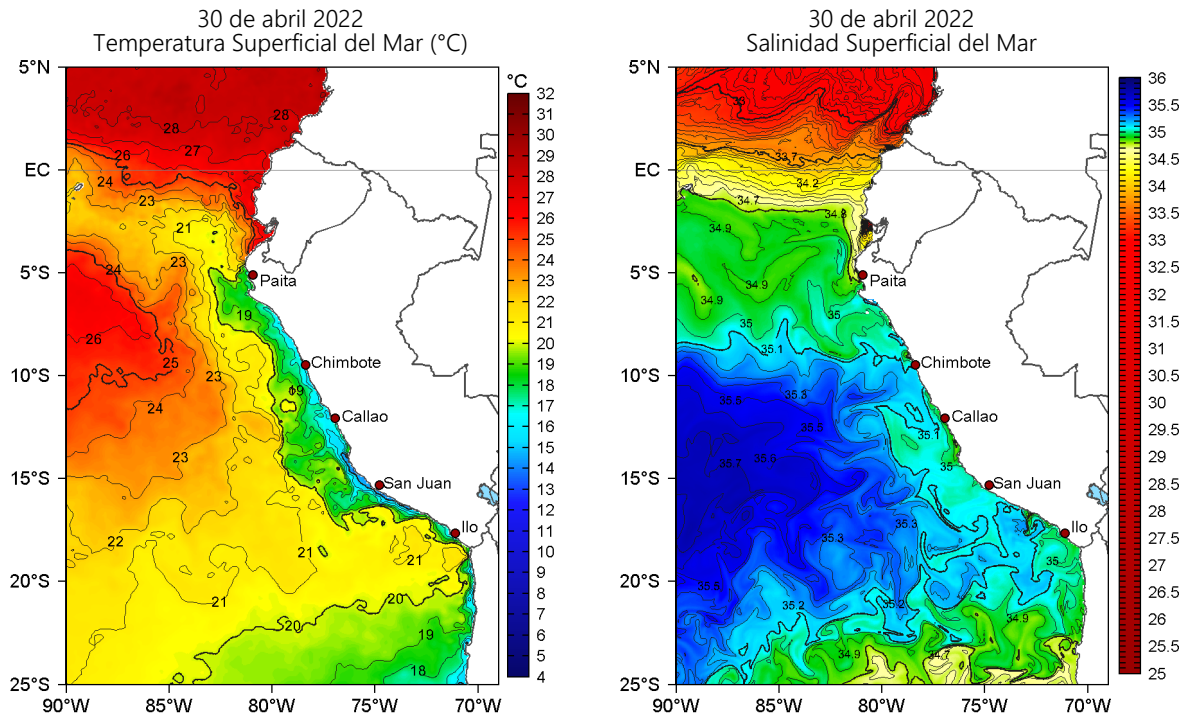
Figura 2. Temperatura superficial del mar (a la izquierda) y Salinidad superficial del mar (a la derecha) para el 30 de abril de 2022. Datos: OSTIA-UKMO-L4-GLOB-v2.0 (UK Met Office, 2012; Donlon et al, 2012) y Hybrid Coordinate Ocean Model v. GOFS 3.1 (HYCOM; Halliwell et al., 1998; 2000; Bleck, 2001), respectivamente.
