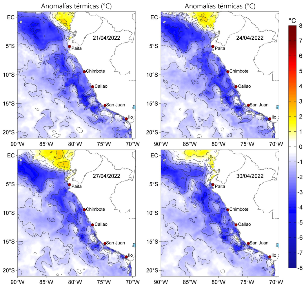
Figura 3. Anomalías de la temperatura superficial del mar (°C) para el 21, 24, 27 y 30 de abril de 2022. Las anomalías se calcularon respecto de la climatología para el periodo 2007-2016. Datos: OSTIA-UKMO-L4-GLOB-v2.0 (UK Met Office, 2012; Donlon et al, 2012).
