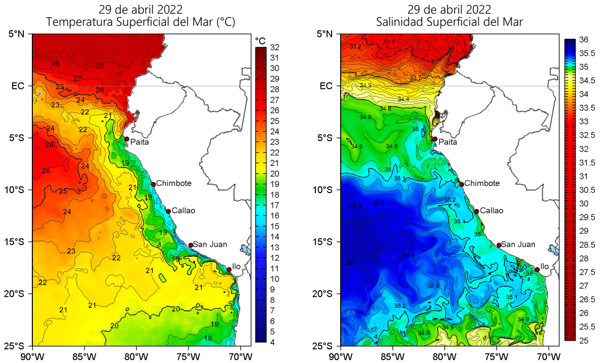
Figura 2. Temperatura superficial del mar (a la izquierda) y Salinidad superficial del mar (a la derecha) para el 29 de abril de 2022. Datos: OSTIA-UKMO-L4-GLOB-v2.0 (UK Met Office, 2012; Donlon et al, 2012) y Hybrid Coordinate Ocean Model v. GOFS 3.1 (HYCOM; Halliwell et al., 1998; 2000; Bleck, 2001), respectivamente.
