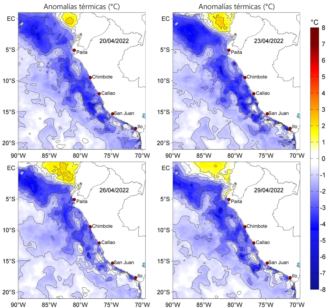
Figura 3. Anomalías de la temperatura superficial del mar (°C) para el 20, 23, 26 y 29 de abril de 2022. Las anomalías se calcularon respecto de la climatología para el periodo 2007-2016. Datos: OSTIA-UKMO-L4-GLOB-v2.0 (UK Met Office, 2012; Donlon et al, 2012).
