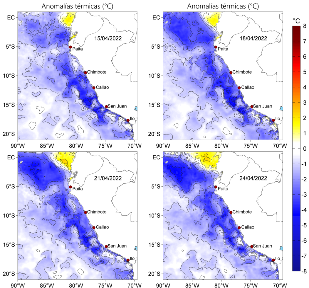
Figura 3. Anomalías de la temperatura superficial del mar (°C) para el 15, 18, 21 y 24 de abril de 2022. Las anomalías se calcularon respecto de la climatología para el periodo 2007-2016. Datos: OSTIA-UKMO-L4-GLOB-v2.0 (UK Met Office, 2012; Donlon et al, 2012).
