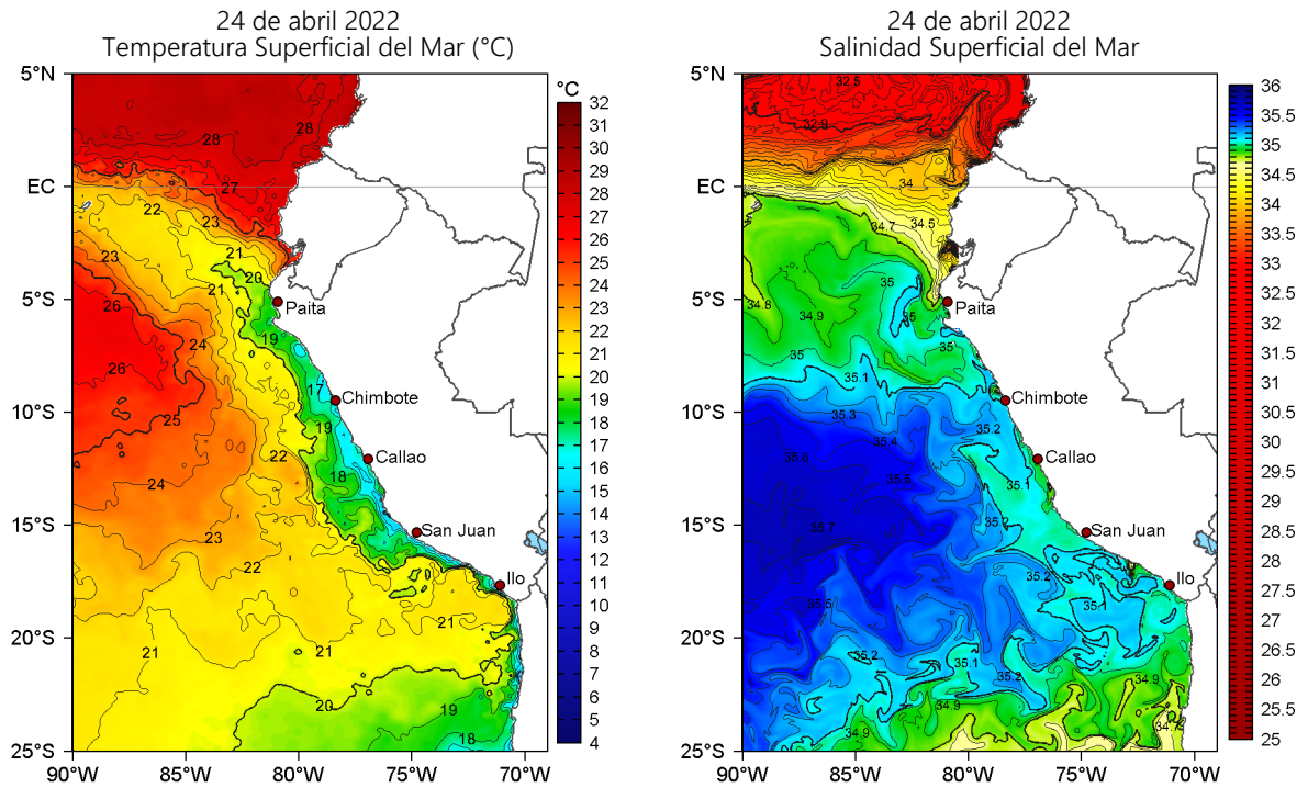
Figura 2. Temperatura superficial del mar (a la izquierda) y Salinidad superficial del mar (a la derecha) para el 24 de abril de 2022. Datos: OSTIA-UKMO-L4-GLOB-v2.0 (UK Met Office, 2012; Donlon et al, 2012) y Hybrid Coordinate Ocean Model v. GOFS 3.1 (HYCOM; Halliwell et al., 1998; 2000; Bleck, 2001), respectivamente.
