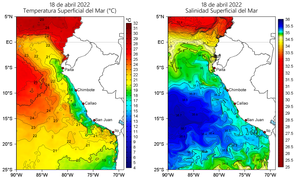
Figura 2. Temperatura superficial del mar (a la izquierda) y Salinidad superficial del mar (a la derecha) para el 18 de abril de 2022. Datos: OSTIA-UKMO-L4-GLOB-v2.0 (UK Met Office, 2012; Donlon et al, 2012) y Hybrid Coordinate Ocean Model v. GOFS 3.1 (HYCOM; Halliwell et al., 1998; 2000; Bleck, 2001), respectivamente.
