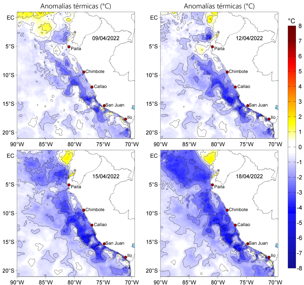
Figura 3. Anomalías de la temperatura superficial del mar (°C) para el 09, 12, 15 y 18 de abril de 2022. Las anomalías se calcularon respecto de la climatología para el periodo 2007-2016. Datos: OSTIA-UKMO-L4-GLOB-v2.0 (UK Met Office, 2012; Donlon et al, 2012).
