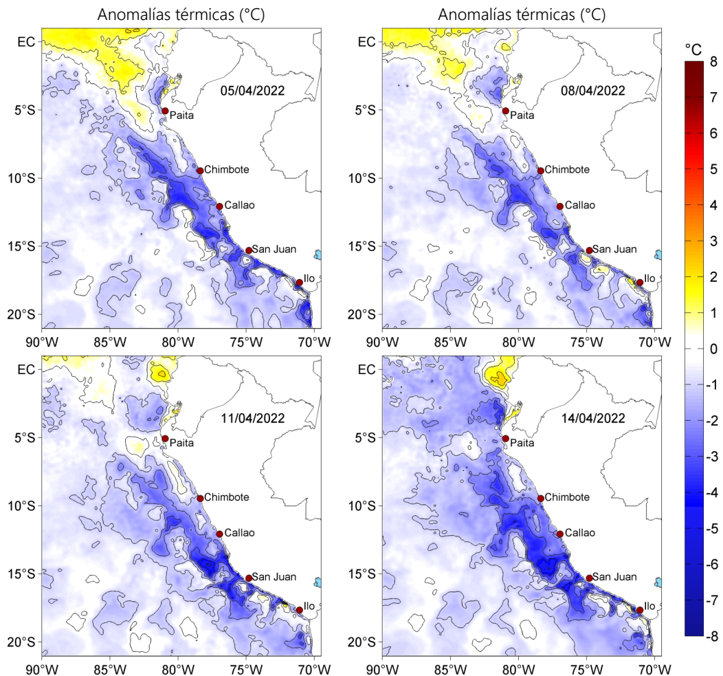
Figura 3. Anomalías de la temperatura superficial del mar (°C) para el 05, 08, 11 y 14 de abril de 2022. Las anomalías se calcularon respecto de la climatología para el periodo 2007-2016. Datos: OSTIA-UKMO-L4-GLOB-v2.0 (UK Met Office, 2012; Donlon et al, 2012).
