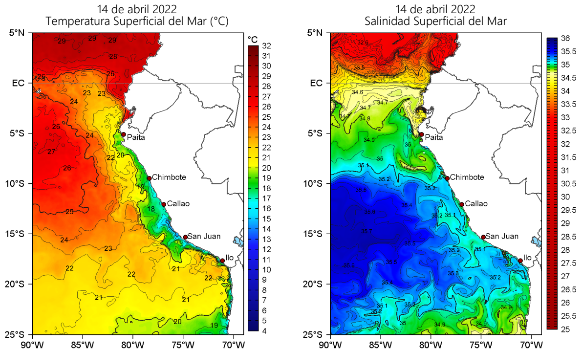
Figura 2. Temperatura superficial del mar (a la izquierda) y Salinidad superficial del mar (a la derecha) para el 14 de abril de 2022. Datos: OSTIA-UKMO-L4-GLOB-v2.0 (UK Met Office, 2012; Donlon et al, 2012) y Hybrid Coordinate Ocean Model v. GOFS 3.1 (HYCOM; Halliwell et al., 1998; 2000; Bleck, 2001), respectivamente.
