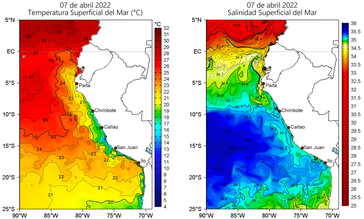
Figura 2. Temperatura superficial del mar (a la izquierda) y Salinidad superficial del mar (a la derecha) para el 07 de abril de 2022. Datos: OSTIA-UKMO-L4-GLOB-v2.0 (UK Met Office, 2012; Donlon et al, 2012) y Hybrid Coordinate Ocean Model v. GOFS 3.1 (HYCOM; Halliwell et al., 1998; 2000; Bleck, 2001), respectivamente.
