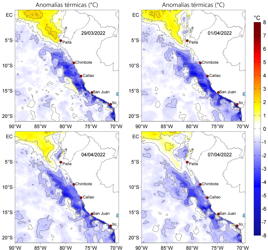
Figura 3. Anomalías de la temperatura superficial del mar (°C) para el 29 de marzo, además del 01, 04 y 07 de abril de 2022. Las anomalías se calcularon respecto de la climatología para el periodo 2007-2016. Datos: OSTIA-UKMO-L4-GLOB-v2.0 (UK Met Office, 2012; Donlon et al, 2012).
