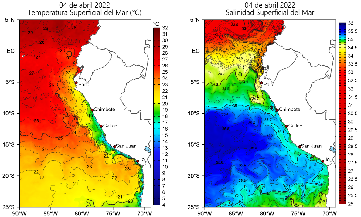
Figura 2. Temperatura superficial del mar (a la izquierda) y Salinidad superficial del mar (a la derecha) para el 04 de abril de 2022. Datos: OSTIA-UKMO-L4-GLOB-v2.0 (UK Met Office, 2012; Donlon et al, 2012) y Hybrid Coordinate Ocean Model v. GOFS 3.1 (HYCOM; Halliwell et al., 1998; 2000; Bleck, 2001), respectivamente.
