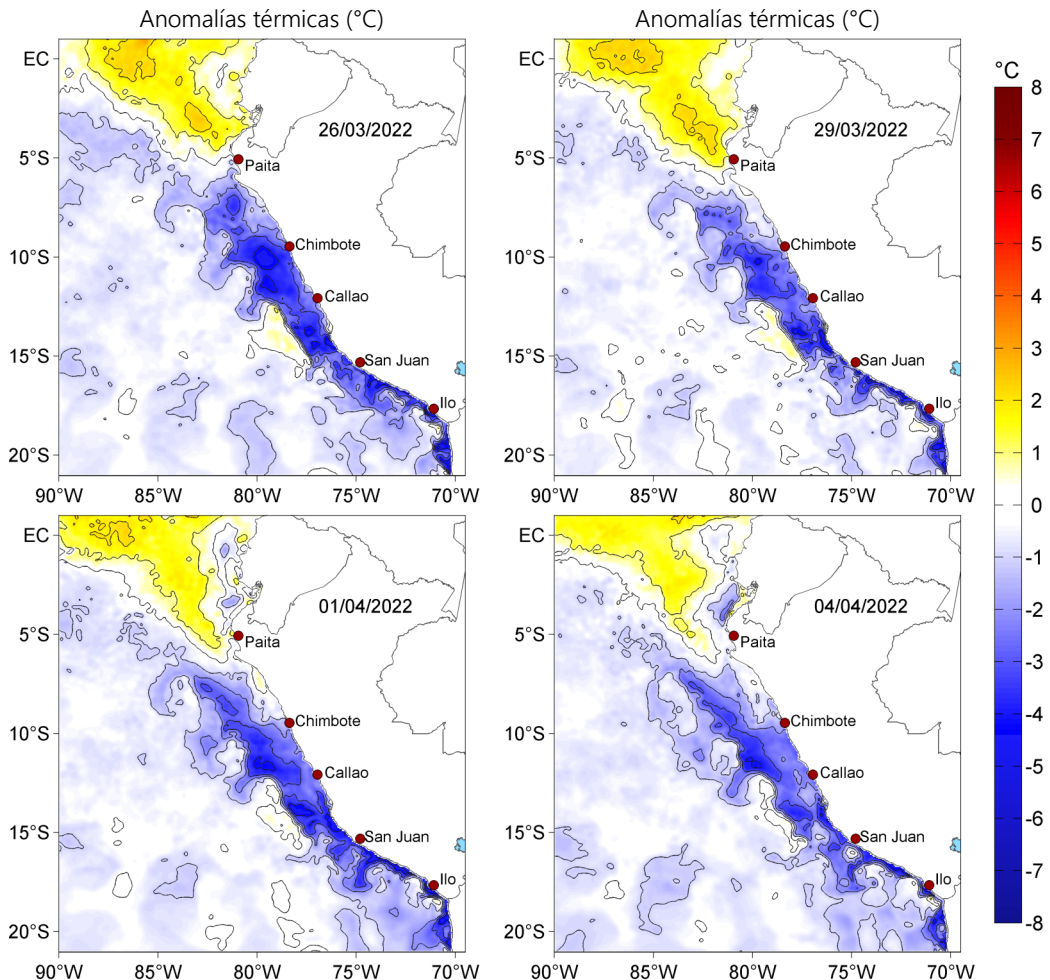
Figura 3. Anomalías de la temperatura superficial del mar (°C) para el 26 y 29 de marzo, además del 01 y 04 de abril de 2022. Las anomalías se calcularon respecto de la climatología para el periodo 2007-2016. Datos: OSTIA-UKMO-L4-GLOB-v2.0 (UK Met Office, 2012; Donlon et al, 2012).
