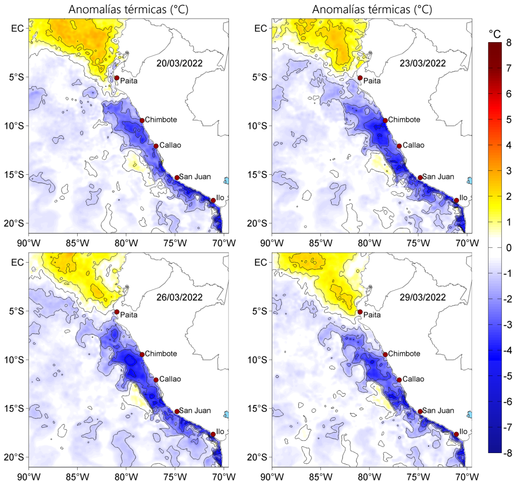
Figura 3. Anomalías de la temperatura superficial del mar (°C) para el 20, 23, 26 y 29 de marzo de 2022. Las anomalías se calcularon respecto de la climatología para el periodo 2007-2016. Datos: OSTIA-UKMO-L4-GLOB-v2.0 (UK Met Office, 2012; Donlon et al, 2012).
