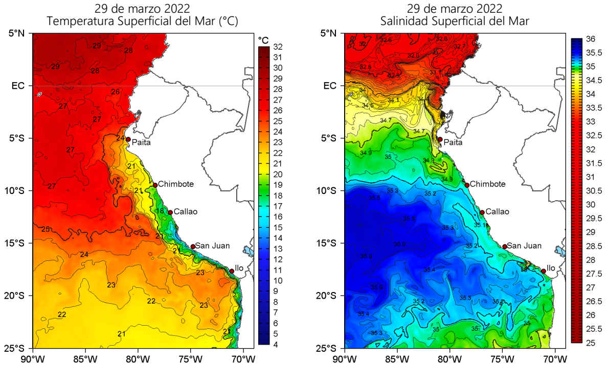
Figura 2. Temperatura superficial del mar (a la izquierda) y Salinidad superficial del mar (a la derecha) para el 29 de marzo de 2022. Datos: OSTIA-UKMO-L4-GLOB-v2.0 (UK Met Office, 2012; Donlon et al, 2012) y Hybrid Coordinate Ocean Model v. GOFS 3.1 (HYCOM; Halliwell et al., 1998; 2000; Bleck, 2001), respectivamente.
