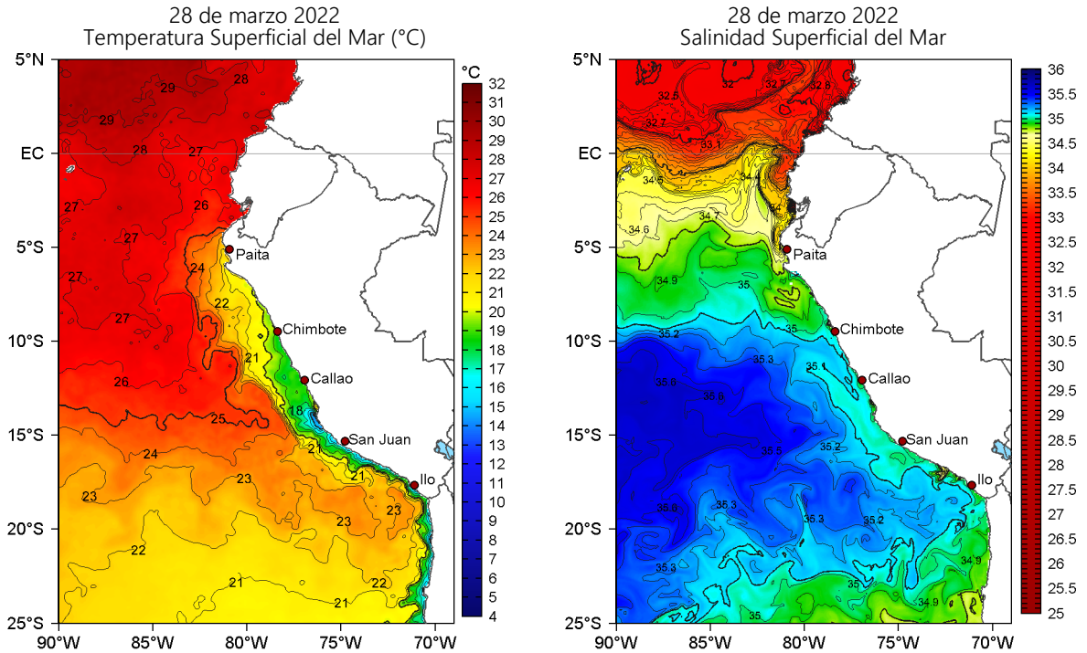
Figura 2. Temperatura superficial del mar (a la izquierda) y Salinidad superficial del mar (a la derecha) para el 28 de marzo de 2022. Datos: OSTIA-UKMO-L4-GLOB-v2.0 (UK Met Office, 2012; Donlon et al, 2012) y Hybrid Coordinate Ocean Model v. GOFS 3.1 (HYCOM; Halliwell et al., 1998; 2000; Bleck, 2001), respectivamente.
