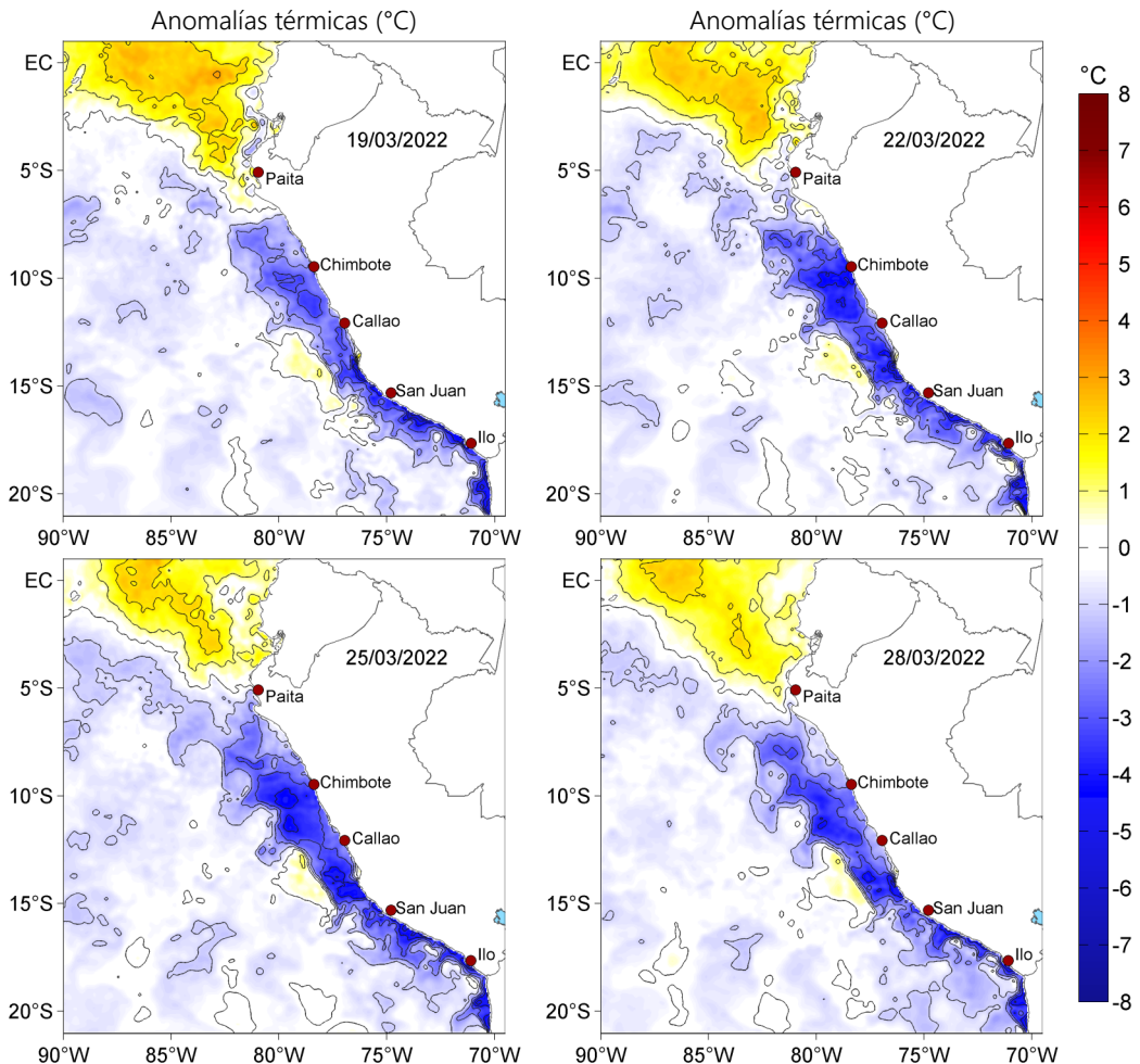
Figura 3. Anomalías de la temperatura superficial del mar (°C) para el 19, 22, 25 y 28 de marzo de 2022. Las anomalías se calcularon respecto de la climatología para el periodo 2007-2016. Datos: OSTIA-UKMO-L4-GLOB-v2.0 (UK Met Office, 2012; Donlon et al, 2012).
