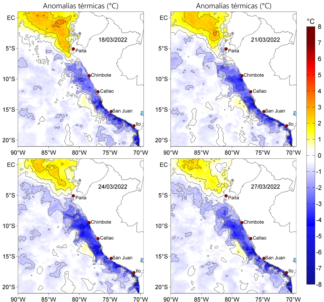
Figura 3. Anomalías de la temperatura superficial del mar (°C) para el 18, 21, 24 y 27 de marzo de 2022. Las anomalías se calcularon respecto de la climatología para el periodo 2007-2016. Datos: OSTIA-UKMO-L4-GLOB-v2.0 (UK Met Office, 2012; Donlon et al, 2012).
