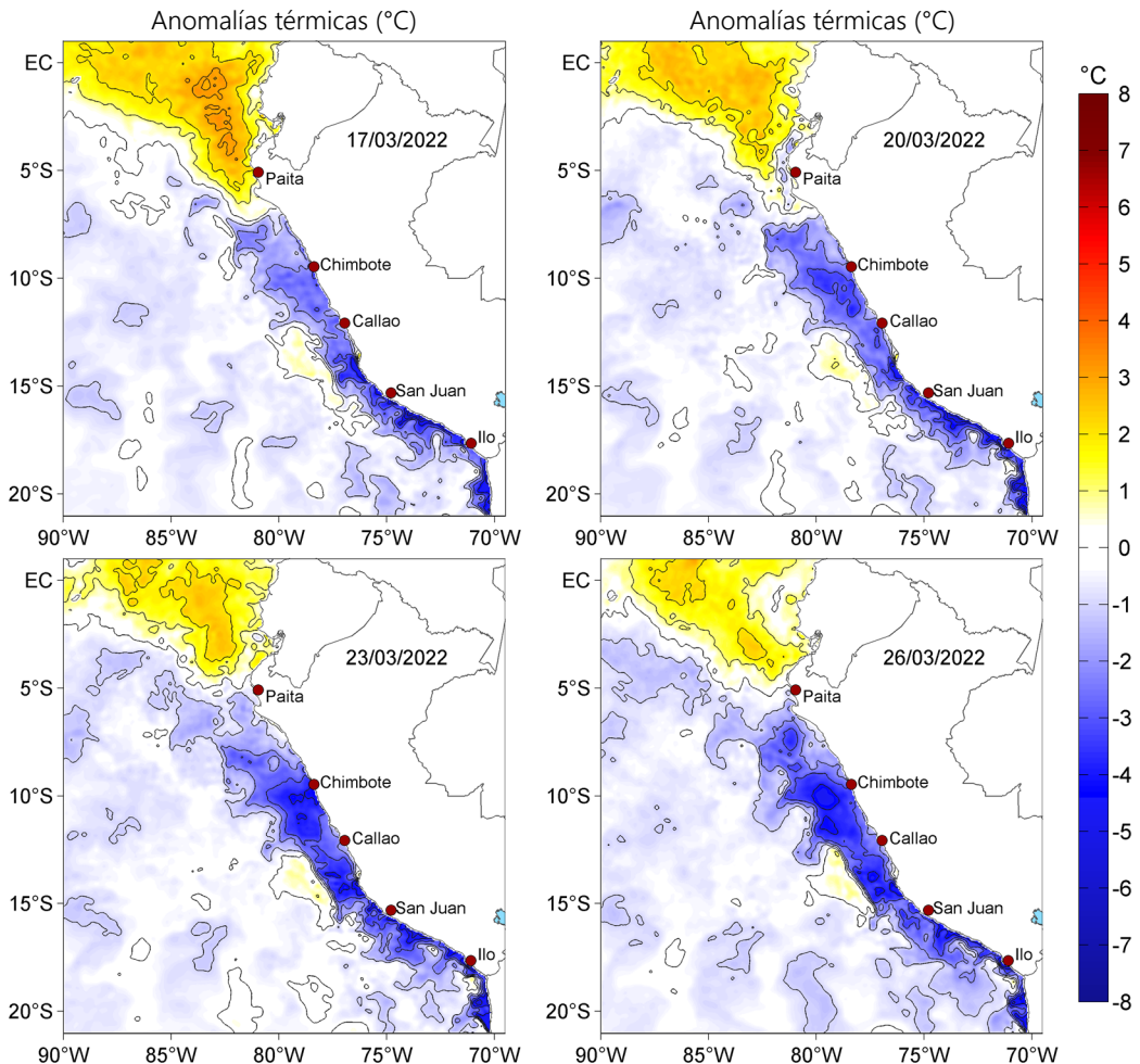
Figura 3. Anomalías de la temperatura superficial del mar (°C) para el 17, 20, 23 y 26 de marzo de 2022. Las anomalías se calcularon respecto de la climatología para el periodo 2007-2016. Datos: OSTIA-UKMO-L4-GLOB-v2.0 (UK Met Office, 2012; Donlon et al, 2012).
