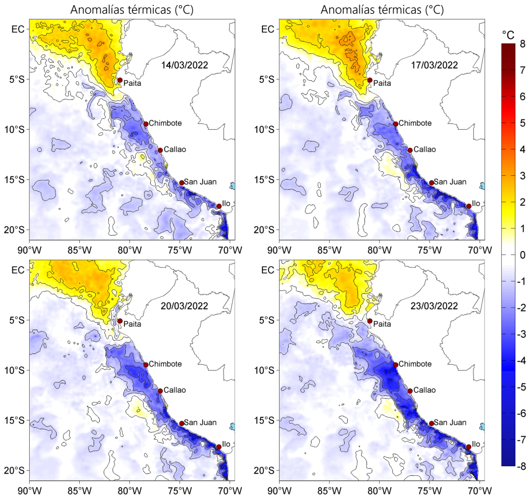
Figura 3. Anomalías de la temperatura superficial del mar (°C) para el 14, 17, 20 y 23 de marzo de 2022. Las anomalías se calcularon respecto de la climatología para el periodo 2007-2016. Datos: OSTIA-UKMO-L4-GLOB-v2.0 (UK Met Office, 2012; Donlon et al, 2012).
