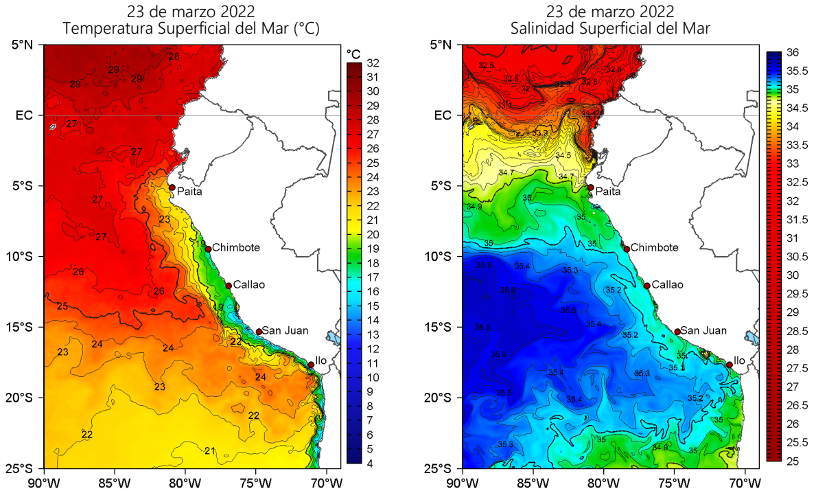
Figura 2. Temperatura superficial del mar (a la izquierda) y Salinidad superficial del mar (a la derecha) para el 23 de marzo de 2022. Datos: OSTIA-UKMO-L4-GLOB-v2.0 (UK Met Office, 2012; Donlon et al, 2012) y Hybrid Coordinate Ocean Model v. GOFS 3.1 (HYCOM; Halliwell et al., 1998; 2000; Bleck, 2001), respectivamente.
