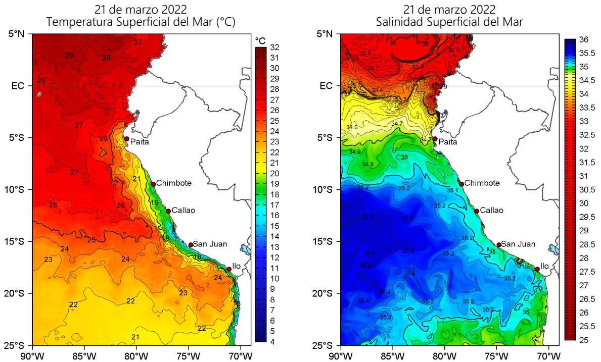
Figura 2. Temperatura superficial del mar (a la izquierda) y Salinidad superficial del mar (a la derecha) para el 21 de marzo de 2022. Datos: OSTIA-UKMO-L4-GLOB-v2.0 (UK Met Office, 2012; Donlon et al, 2012) y Hybrid Coordinate Ocean Model v. GOFS 3.1 (HYCOM; Halliwell et al., 1998; 2000; Bleck, 2001), respectivamente.
