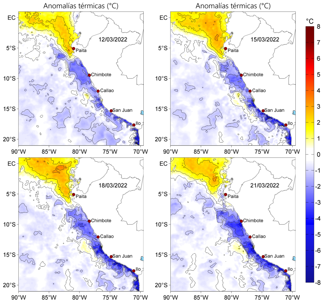
Figura 3. Anomalías de la temperatura superficial del mar (°C) para el 12, 15, 18 y 21 de marzo de 2022. Las anomalías se calcularon respecto de la climatología para el periodo 2007-2016. Datos: OSTIA-UKMO-L4-GLOB-v2.0 (UK Met Office, 2012; Donlon et al, 2012).
