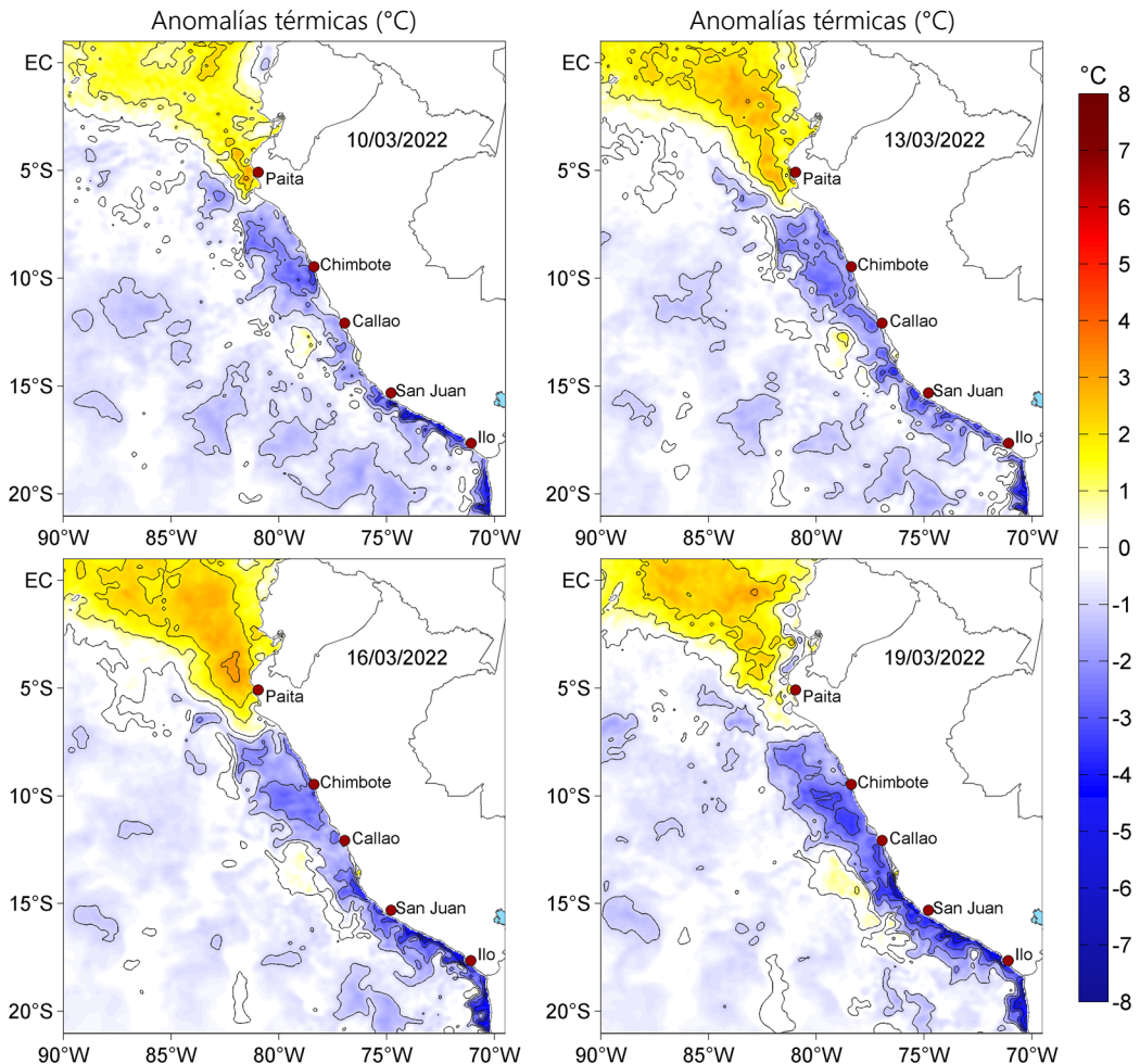
Figura 3. Anomalías de la temperatura superficial del mar (°C) para el 10, 13, 16 y 19 de marzo de 2022. Las anomalías se calcularon respecto de la climatología para el periodo 2007-2016. Datos: OSTIA-UKMO-L4-GLOB-v2.0 (UK Met Office, 2012; Donlon et al, 2012).
