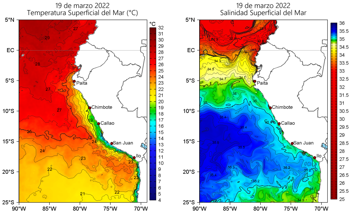
Figura 2. Temperatura superficial del mar (a la izquierda) y Salinidad superficial del mar (a la derecha) para el 19 de marzo de 2022. Datos: OSTIA-UKMO-L4-GLOB-v2.0 (UK Met Office, 2012; Donlon et al, 2012) y Hybrid Coordinate Ocean Model v. GOFS 3.1 (HYCOM; Halliwell et al., 1998; 2000; Bleck, 2001), respectivamente.
