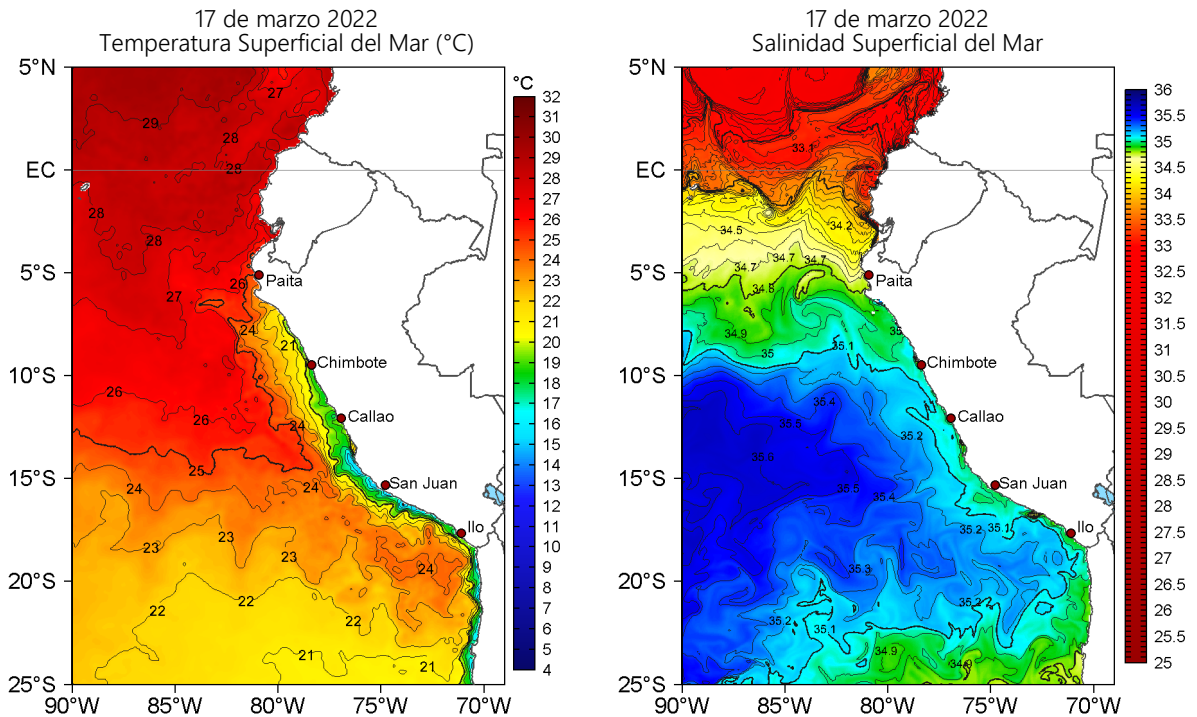
Figura 2. Temperatura superficial del mar (a la izquierda) y Salinidad superficial del mar (a la derecha) para el 17 de marzo de 2022. Datos: OSTIA-UKMO-L4-GLOB-v2.0 (UK Met Office, 2012; Donlon et al, 2012) y Hybrid Coordinate Ocean Model v. GOFS 3.1 (HYCOM; Halliwell et al., 1998; 2000; Bleck, 2001), respectivamente.
