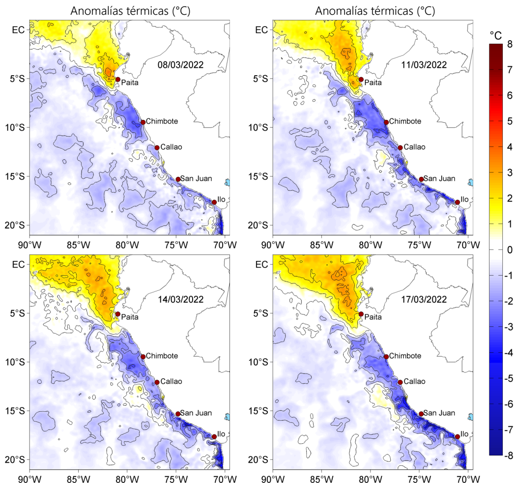
Figura 3. Anomalías de la temperatura superficial del mar (°C) para el 08, 11, 14 y 17 de marzo de 2022. Las anomalías se calcularon respecto de la climatología para el periodo 2007-2016. Datos: OSTIA-UKMO-L4-GLOB-v2.0 (UK Met Office, 2012; Donlon et al, 2012).
