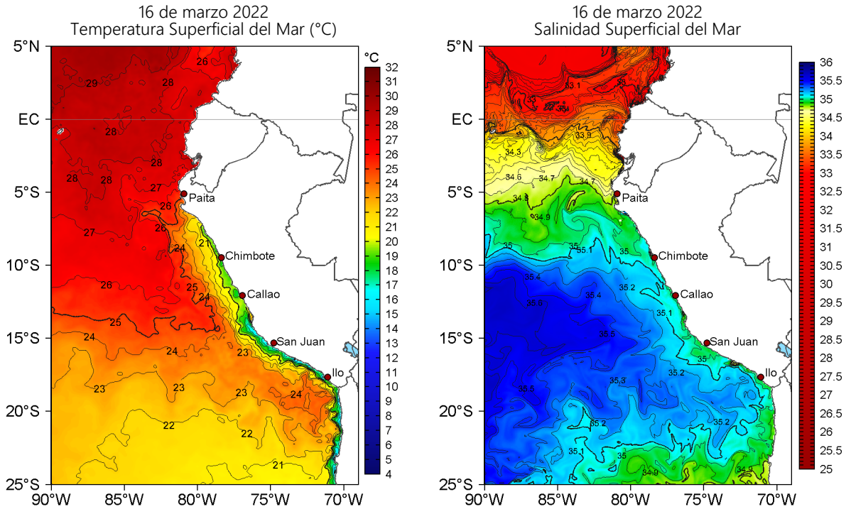
Figura 2. Temperatura superficial del mar (a la izquierda) y Salinidad superficial del mar (a la derecha) para el 16 de marzo de 2022. Datos: OSTIA-UKMO-L4-GLOB-v2.0 (UK Met Office, 2012; Donlon et al, 2012) y Hybrid Coordinate Ocean Model v. GOFS 3.1 (HYCOM; Halliwell et al., 1998; 2000; Bleck, 2001), respectivamente.
