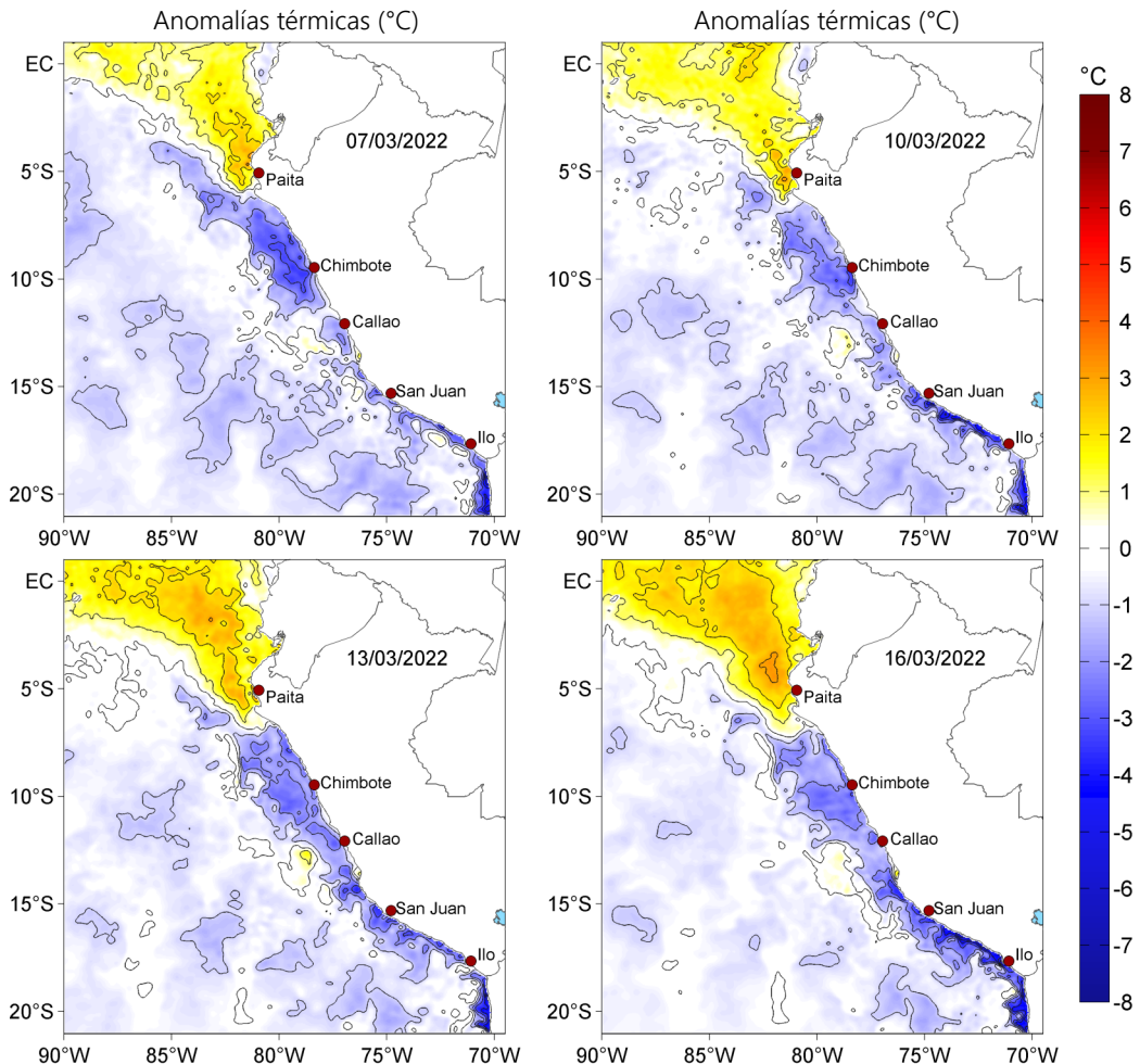
Figura 3. Anomalías de la temperatura superficial del mar (°C) para el 07, 10, 13 y 16 de marzo de 2022. Las anomalías se calcularon respecto de la climatología para el periodo 2007-2016. Datos: OSTIA-UKMO-L4-GLOB-v2.0 (UK Met Office, 2012; Donlon et al, 2012).
