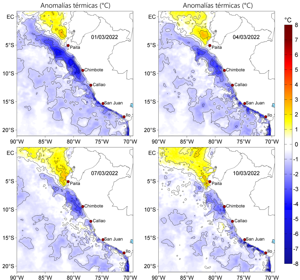
Figura 3. Anomalías de la temperatura superficial del mar (°C) para el 01, 04, 07 y 10 de marzo de 2022. Las anomalías se calcularon respecto de la climatología para el periodo 2007-2016. Datos: OSTIA-UKMO-L4-GLOB-v2.0 (UK Met Office, 2012; Donlon et al, 2012).
