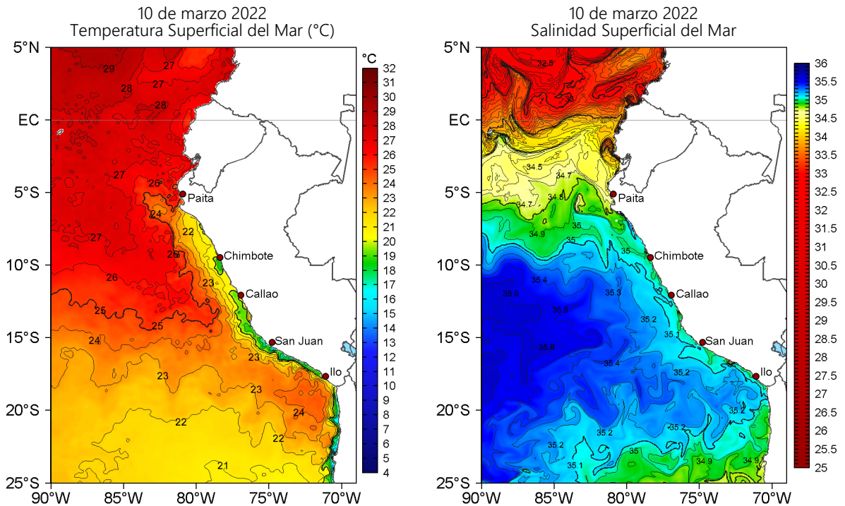
Figura 2. Temperatura superficial del mar (a la izquierda) y Salinidad superficial del mar (a la derecha) para el 10 de marzo de 2022. Datos: OSTIA-UKMO-L4-GLOB-v2.0 (UK Met Office, 2012; Donlon et al, 2012) y Hybrid Coordinate Ocean Model v. GOFS 3.1 (HYCOM; Halliwell et al., 1998; 2000; Bleck, 2001), respectivamente.
