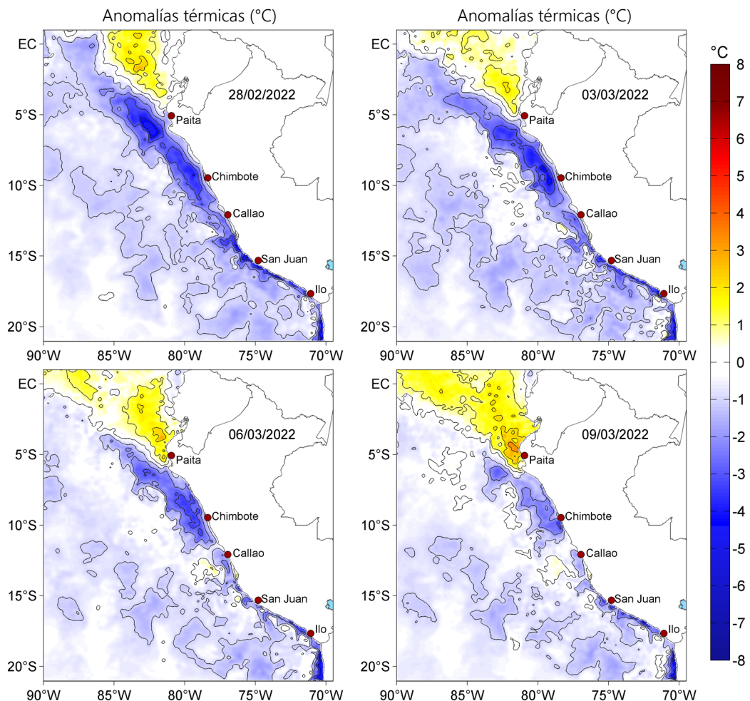
Figura 3. Anomalías de la temperatura superficial del mar (°C) para el 28 de febrero, así como para el 03, 06 y 09 de marzo de 2022. Las anomalías se calcularon respecto de la climatología para el periodo 2007-2016. Datos: OSTIA-UKMO-L4-GLOB-v2.0 (UK Met Office, 2012; Donlon et al, 2012).
