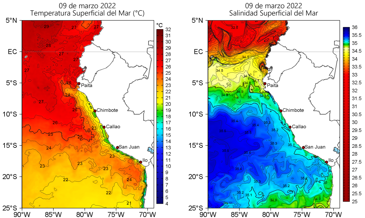
Figura 2. Temperatura superficial del mar (a la izquierda) y Salinidad superficial del mar (a la derecha) para el 09 de marzo de 2022. Datos: OSTIA-UKMO-L4-GLOB-v2.0 (UK Met Office, 2012; Donlon et al, 2012) y Hybrid Coordinate Ocean Model v. GOFS 3.1 (HYCOM; Halliwell et al., 1998; 2000; Bleck, 2001), respectivamente.
