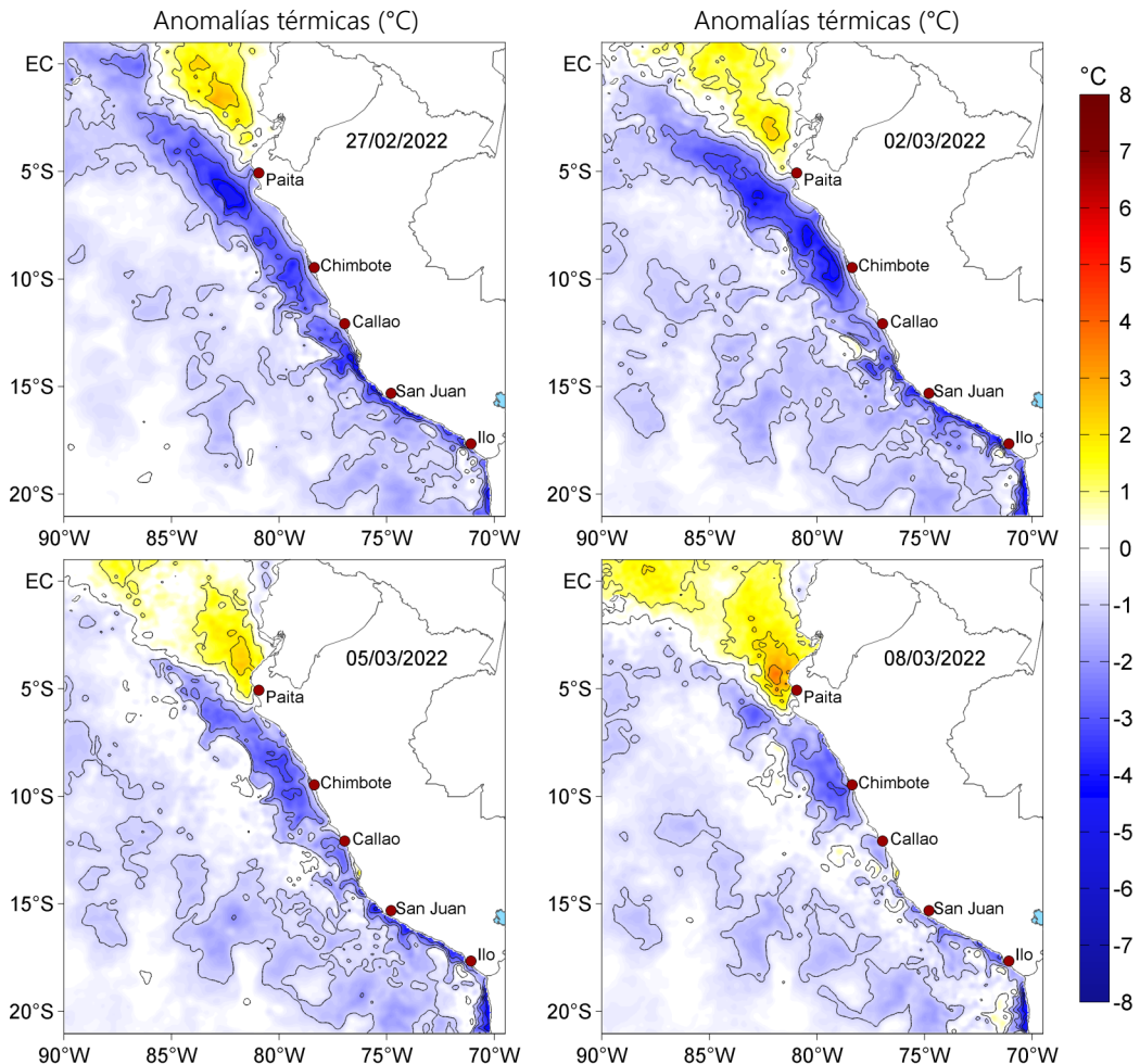
Figura 3. Anomalías de la temperatura superficial del mar (°C) para el 27 de febrero, así como para el 02, 05 y 08 de marzo de 2022. Las anomalías se calcularon respecto de la climatología para el periodo 2007-2016. Datos: OSTIA-UKMO-L4-GLOB-v2.0 (UK Met Office, 2012; Donlon et al, 2012).
