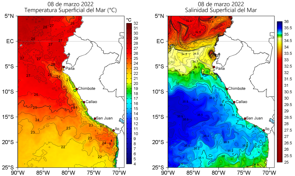
Figura 2. Temperatura superficial del mar (a la izquierda) y Salinidad superficial del mar (a la derecha) para el 08 de marzo de 2022. Datos: OSTIA-UKMO-L4-GLOB-v2.0 (UK Met Office, 2012; Donlon et al, 2012) y Hybrid Coordinate Ocean Model v. GOFS 3.1 (HYCOM; Halliwell et al., 1998; 2000; Bleck, 2001), respectivamente.
