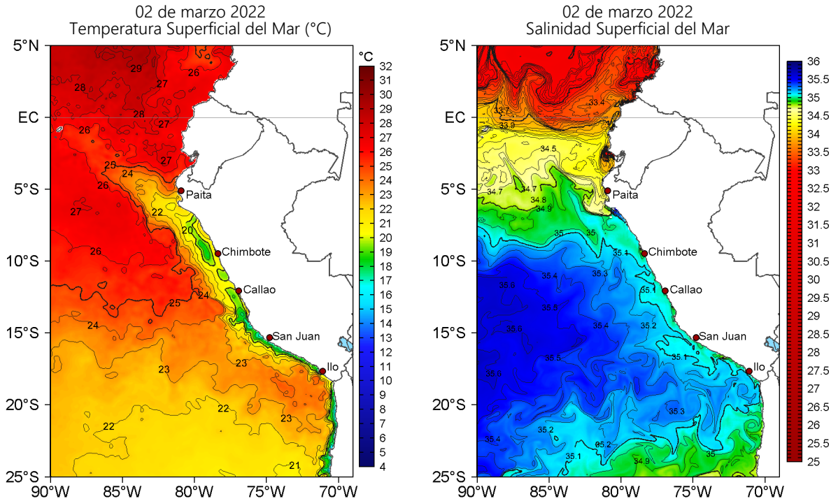
Figura 2. Temperatura superficial del mar (a la izquierda) y Salinidad superficial del mar (a la derecha) para el 02 de marzo de 2022. Datos: OSTIA-UKMO-L4-GLOB-v2.0 (UK Met Office, 2012; Donlon et al, 2012) y Hybrid Coordinate Ocean Model v. GOFS 3.1 (HYCOM; Halliwell et al., 1998; 2000; Bleck, 2001), respectivamente.
