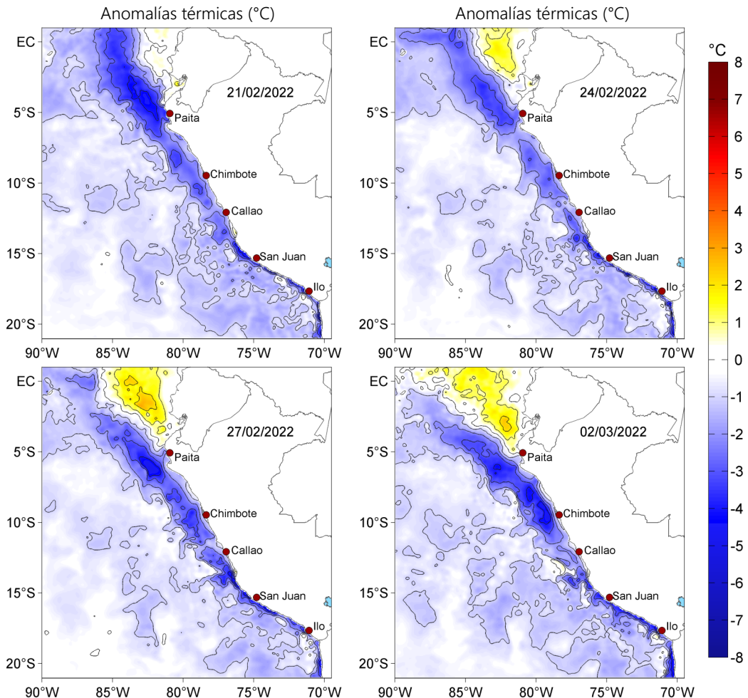
Figura 3. Anomalías de la temperatura superficial del mar (°C) para los días 21, 24 y 27 de febrero, así como para el 02 de marzo de 2022. Las anomalías se calcularon respecto de la climatología para el periodo 2007-2016. Datos: OSTIA-UKMO-L4-GLOB-v2.0 (UK Met Office, 2012; Donlon et al, 2012).
