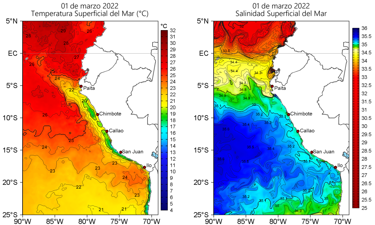
Figura 2. Temperatura superficial del mar (a la izquierda) y Salinidad superficial del mar (a la derecha) para el 01 de marzo de 2022. Datos: OSTIA-UKMO-L4-GLOB-v2.0 (UK Met Office, 2012; Donlon et al, 2012) y Hybrid Coordinate Ocean Model v. GOFS 3.1 (HYCOM; Halliwell et al., 1998; 2000; Bleck, 2001), respectivamente.
