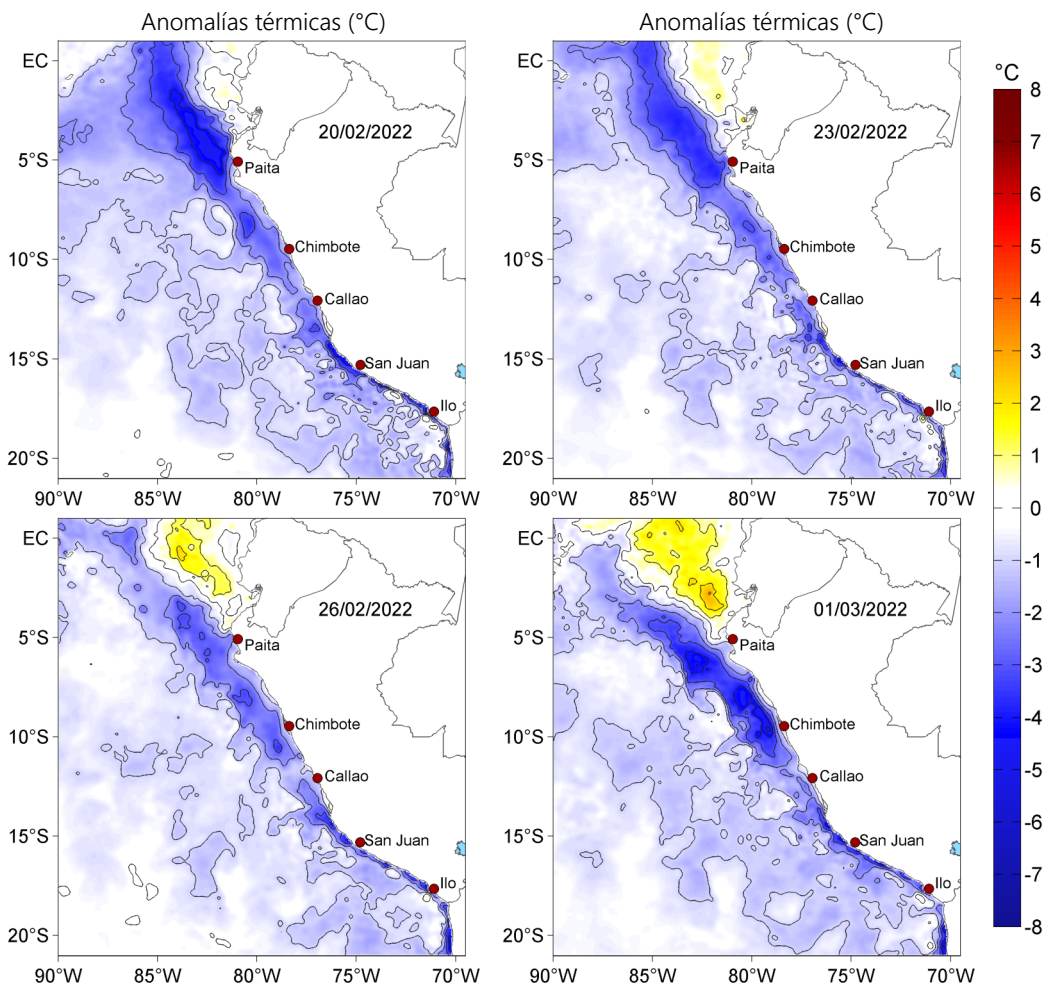
Figura 3. Anomalías de la temperatura superficial del mar (°C) para los días 20, 23 y 26 de febrero, así como para el 01 de marzo de 2022. Las anomalías se calcularon respecto de la climatología para el periodo 2007-2016. Datos: OSTIA-UKMO-L4-GLOB-v2.0 (UK Met Office, 2012; Donlon et al, 2012).
