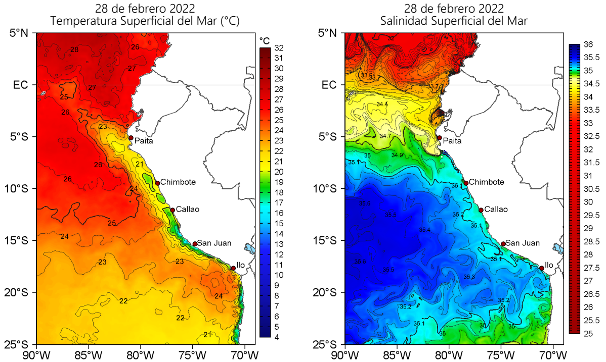
Figura 2. Temperatura superficial del mar (a la izquierda) y Salinidad superficial del mar (a la derecha) para el 28 de febrero de 2022. Datos: OSTIA-UKMO-L4-GLOB-v2.0 (UK Met Office, 2012; Donlon et al, 2012) y Hybrid Coordinate Ocean Model v. GOFS 3.1 (HYCOM; Halliwell et al., 1998; 2000; Bleck, 2001), respectivamente.
