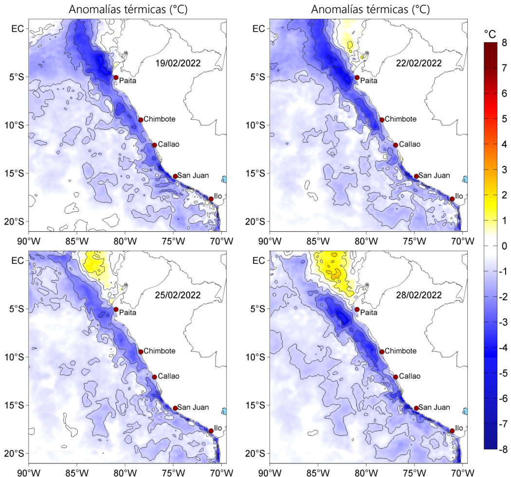
Figura 3. Anomalías de la temperatura superficial del mar (°C) para el 19, 22, 25 y 28 de febrero de 2022. Las anomalías se calcularon respecto de la climatología para el periodo 2007-2016. Datos: OSTIA-UKMO-L4-GLOB-v2.0 (UK Met Office, 2012; Donlon et al, 2012).
