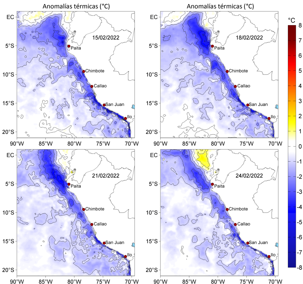
Figura 3. Anomalías de la temperatura superficial del mar (°C) para el 15, 18, 21 y 24 de febrero de 2022. Las anomalías se calcularon respecto de la climatología para el periodo 2007-2016. Datos: OSTIA-UKMO-L4-GLOB-v2.0 (UK Met Office, 2012; Donlon et al, 2012).
