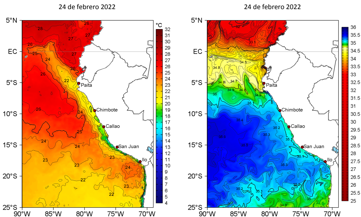
Figura 2. Temperatura superficial del mar (a la izquierda) y Salinidad superficial del mar (a la derecha) para el 24 de febrero de 2022. Datos: OSTIA-UKMO-L4-GLOB-v2.0 (UK Met Office, 2012; Donlon et al, 2012) y Hybrid Coordinate Ocean Model v. GOFS 3.1 (HYCOM; Halliwell et al., 1998; 2000; Bleck, 2001), respectivamente.
