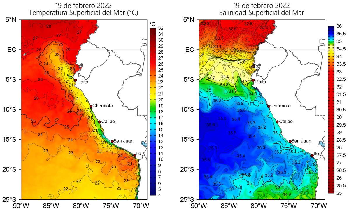
Figura 2. Temperatura superficial del mar (a la izquierda) y Salinidad superficial del mar (a la derecha) para el 19 de febrero de 2022. Datos: OSTIA-UKMO-L4-GLOB-v2.0 (UK Met Office, 2012; Donlon et al, 2012) y Hybrid Coordinate Ocean Model v. GOFS 3.1 (HYCOM; Halliwell et al., 1998; 2000; Bleck, 2001), respectivamente.
