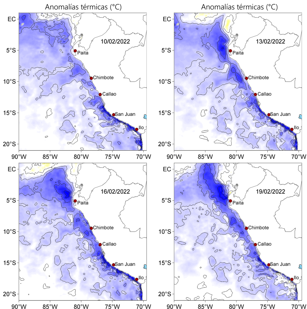
Figura 3. Anomalías de la temperatura superficial del mar (°C) para el 10, 13, 16 y 19 de febrero de 2022. Las anomalías se calcularon respecto de la climatología para el periodo 2007-2016. Datos: OSTIA-UKMO-L4-GLOB-v2.0 (UK Met Office, 2012; Donlon et al, 2012).
