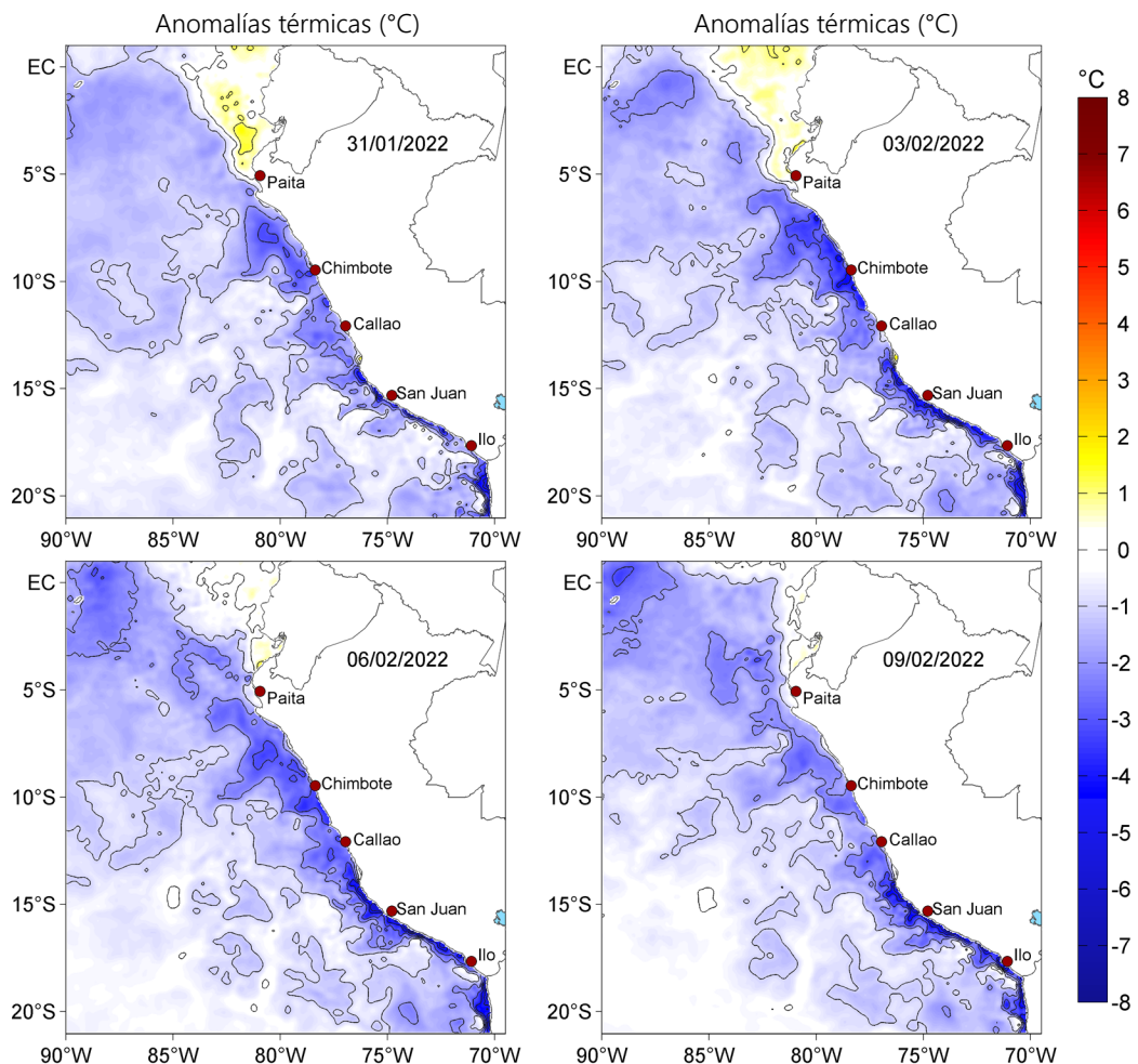
Figura 3. Anomalías de la temperatura superficial del mar (°C) para el 31 de enero, así como para el 03, 06 y 09 de febrero de 2022. Las anomalías se calcularon respecto de la climatología para el periodo 2007-2016. Datos: OSTIA-UKMO-L4-GLOB-v2.0 (UK Met Office, 2012; Donlon et al, 2012).
