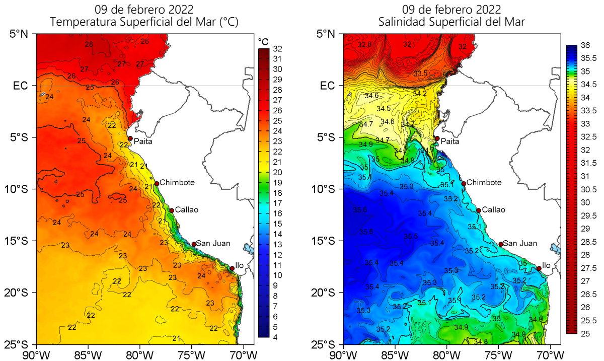
Figura 2. Temperatura superficial del mar (a la izquierda) y Salinidad superficial del mar (a la derecha) para el 09 de febrero de 2022. Datos: OSTIA-UKMO-L4-GLOB-v2.0 (UK Met Office, 2012; Donlon et al, 2012) y Hybrid Coordinate Ocean Model v. GOFS 3.1 (HYCOM; Halliwell et al., 1998; 2000; Bleck, 2001), respectivamente.
