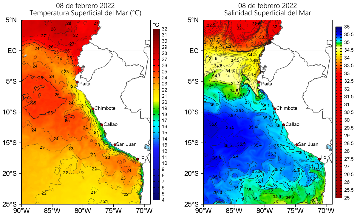
Figura 2. Temperatura superficial del mar (a la izquierda) y Salinidad superficial del mar (a la derecha) para el 08 de febrero de 2022. Datos: OSTIA-UKMO-L4-GLOB-v2.0 (UK Met Office, 2012; Donlon et al, 2012) y Hybrid Coordinate Ocean Model v. GOFS 3.1 (HYCOM; Halliwell et al., 1998; 2000; Bleck, 2001), respectivamente.
