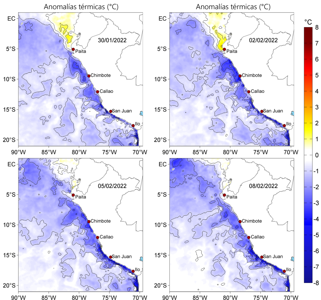
Figura 3. Anomalías de la temperatura superficial del mar (°C) para el 30 de enero, así como para el 02, 05 y 08 de febrero de 2022. Las anomalías se calcularon respecto de la climatología para el periodo 2007-2016. Datos: OSTIA-UKMO-L4-GLOB-v2.0 (UK Met Office, 2012; Donlon et al, 2012).
