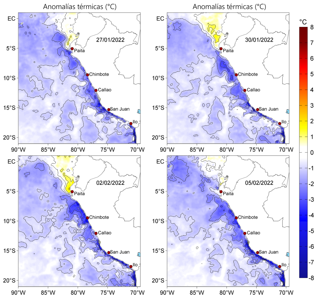
Figura 3. Anomalías de la temperatura superficial del mar (°C) para los días 27 y 30 de enero, así como para el 02 y 05 de febrero de 2022. Las anomalías se calcularon respecto de la climatología para el periodo 2007-2016. Datos: OSTIA-UKMO-L4-GLOB-v2.0 (UK Met Office, 2012; Donlon et al, 2012).
