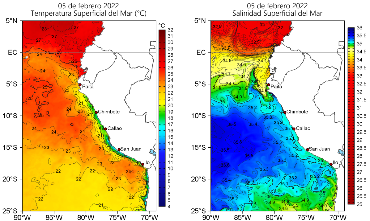
Figura 2. Temperatura superficial del mar (a la izquierda) y Salinidad superficial del mar (a la derecha) para el 05 de febrero de 2022. Datos: OSTIA-UKMO-L4-GLOB-v2.0 (UK Met Office, 2012; Donlon et al, 2012) y Hybrid Coordinate Ocean Model v. GOFS 3.1 (HYCOM; Halliwell et al., 1998; 2000; Bleck, 2001), respectivamente.
