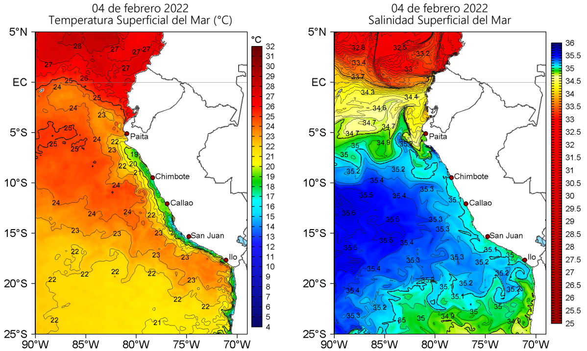
Figura 2. Temperatura superficial del mar (a la izquierda) y Salinidad superficial del mar (a la derecha) para el 04 de febrero de 2022. Datos: OSTIA-UKMO-L4-GLOB-v2.0 (UK Met Office, 2012; Donlon et al, 2012) y Hybrid Coordinate Ocean Model v. GOFS 3.1 (HYCOM; Halliwell et al., 1998; 2000; Bleck, 2001), respectivamente.
