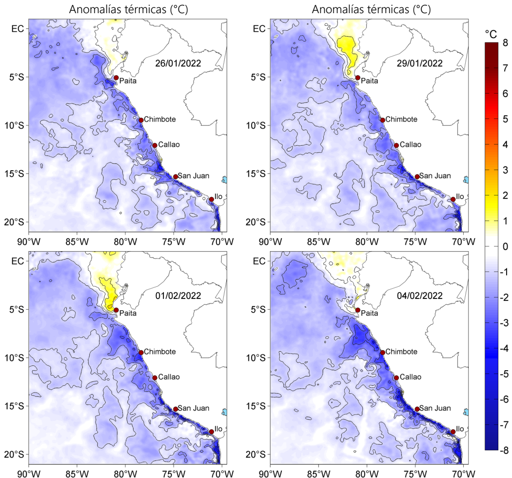
Figura 3. Anomalías de la temperatura superficial del mar (°C) para los días 26 y 29 de enero, así como para el 01 y 04 de febrero de 2022. Las anomalías se calcularon respecto de la climatología para el periodo 2007-2016. Datos: OSTIA-UKMO-L4-GLOB-v2.0 (UK Met Office, 2012; Donlon et al, 2012).
