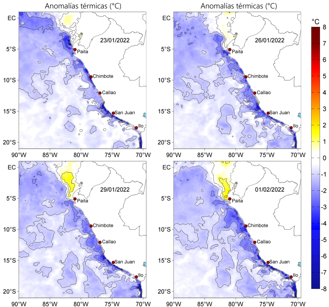
Figura 3. Anomalías de la temperatura superficial del mar (°C) para los días 23, 26 y 29 de enero, así como para el 01 de febrero de 2022. Las anomalías se calcularon respecto de la climatología para el periodo 2007-2016. Datos: OSTIA-UKMO-L4-GLOB-v2.0 (UK Met Office, 2012; Donlon et al, 2012).
