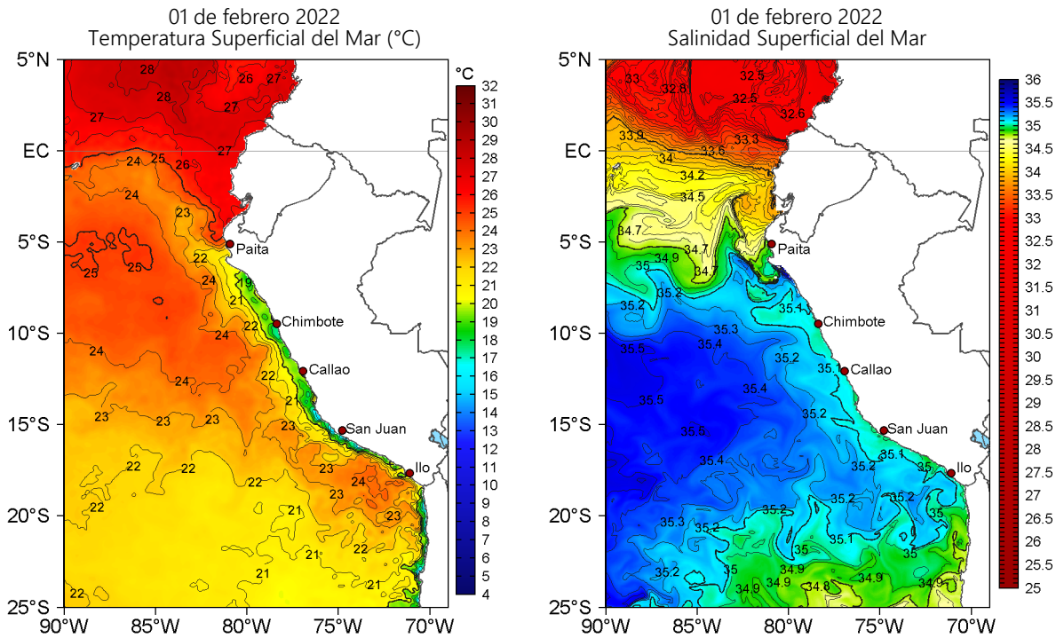
Figura 2. Temperatura superficial del mar (a la izquierda) y Salinidad superficial del mar (a la derecha) para el 01 de febrero de 2022. Datos: OSTIA-UKMO-L4-GLOB-v2.0 (UK Met Office, 2012; Donlon et al, 2012) y Hybrid Coordinate Ocean Model v. GOFS 3.1 (HYCOM; Halliwell et al., 1998; 2000; Bleck, 2001), respectivamente.
