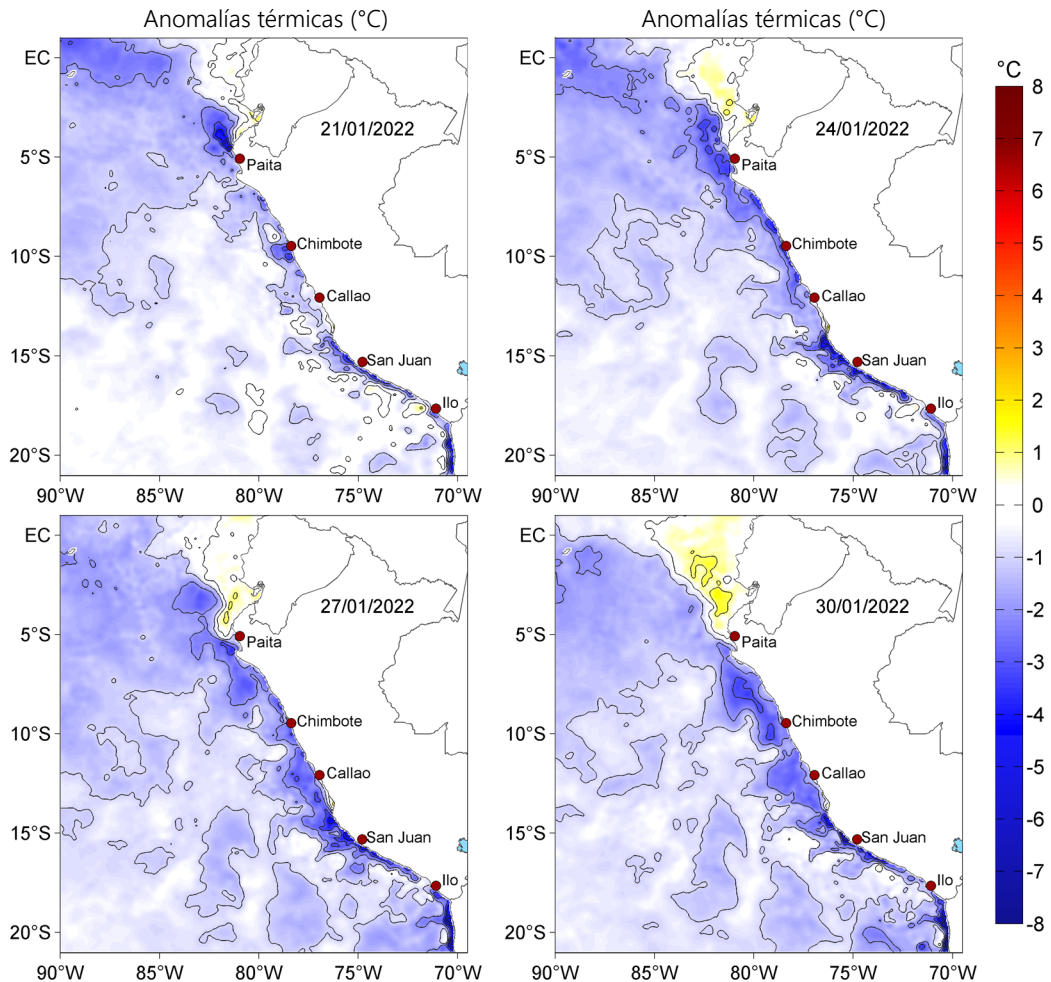
Figura 3. Anomalías de la temperatura superficial del mar (°C) para el 21, 24, 27 y 30 de enero de 2022. Las anomalías se calcularon respecto de la climatología para el periodo 2007-2016. Datos: OSTIA-UKMO-L4-GLOB-v2.0 (UK Met Office, 2012; Donlon et al, 2012).
