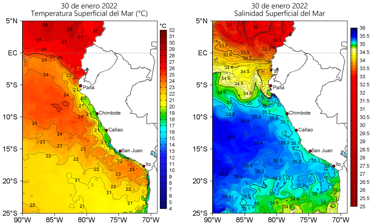
Figura 2. Temperatura superficial del mar (a la izquierda) y Salinidad superficial del mar (a la derecha) para el 30 de enero de 2022. Datos: OSTIA-UKMO-L4-GLOB-v2.0 (UK Met Office, 2012; Donlon et al, 2012) y Hybrid Coordinate Ocean Model v. GOFS 3.1 (HYCOM; Halliwell et al., 1998; 2000; Bleck, 2001), respectivamente.
