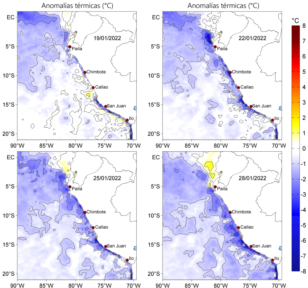
Figura 3. Anomalías de la temperatura superficial del mar (°C) para el 19, 22, 25 y 28 de enero de 2022. Las anomalías se calcularon respecto de la climatología para el periodo 2007-2016. Datos: OSTIA-UKMO-L4-GLOB-v2.0 (UK Met Office, 2012; Donlon et al, 2012).
