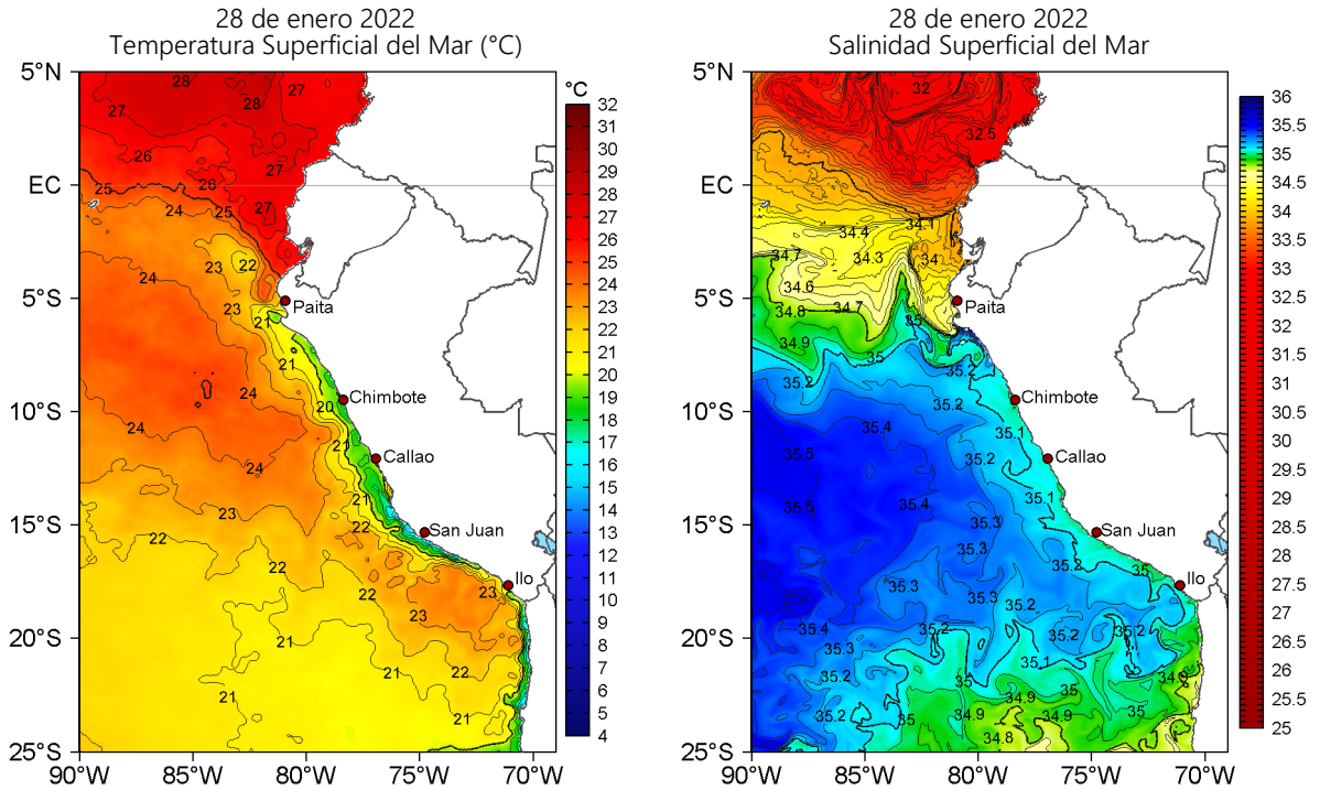
Figura 2. Temperatura superficial del mar (a la izquierda) y Salinidad superficial del mar (a la derecha) para el 28 de enero de 2022. Datos: OSTIA-UKMO-L4-GLOB-v2.0 (UK Met Office, 2012; Donlon et al, 2012) y Hybrid Coordinate Ocean Model v. GOFS 3.1 (HYCOM; Halliwell et al., 1998; 2000; Bleck, 2001), respectivamente.
