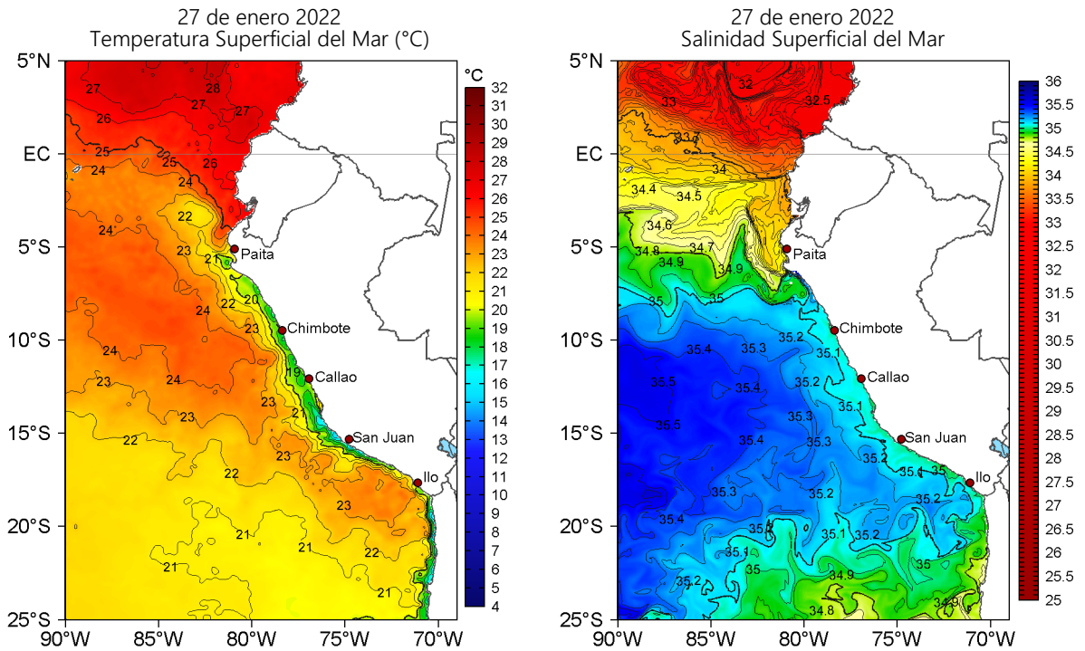
Figura 2. Temperatura superficial del mar (a la izquierda) y Salinidad superficial del mar (a la derecha) para el 27 de enero de 2022. Datos: OSTIA-UKMO-L4-GLOB-v2.0 (UK Met Office, 2012; Donlon et al, 2012) y Hybrid Coordinate Ocean Model v. GOFS 3.1 (HYCOM; Halliwell et al., 1998; 2000; Bleck, 2001), respectivamente.
