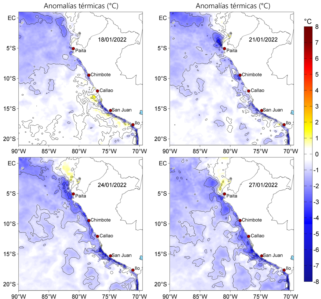
Figura 3. Anomalías de la temperatura superficial del mar (°C) para el 18, 21, 24 y 27 de enero de 2022. Las anomalías se calcularon respecto de la climatología para el periodo 2007-2016. Datos: OSTIA-UKMO-L4-GLOB-v2.0 (UK Met Office, 2012; Donlon et al, 2012).
