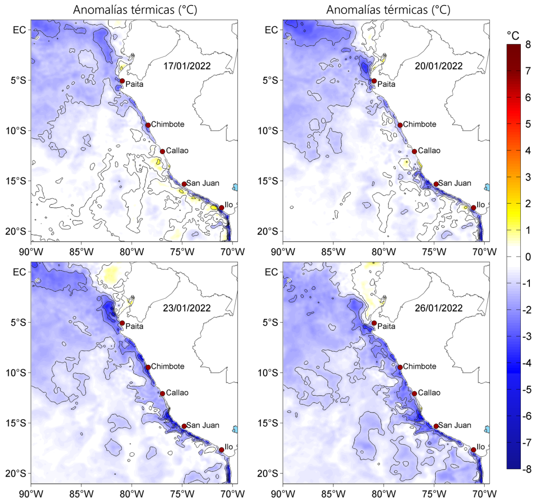
Figura 3. Anomalías de la temperatura superficial del mar (°C) para el 17, 20, 23 y 26 de enero de 2022. Las anomalías se calcularon respecto de la climatología para el periodo 2007-2016. Datos: OSTIA-UKMO-L4-GLOB-v2.0 (UK Met Office, 2012; Donlon et al, 2012).
