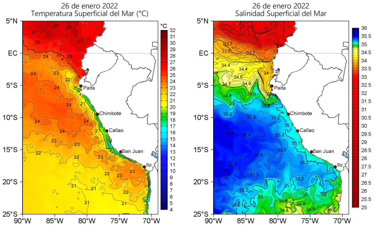
Figura 2. Temperatura superficial del mar (a la izquierda) y Salinidad superficial del mar (a la derecha) para el 26 de enero de 2022. Datos: OSTIA-UKMO-L4-GLOB-v2.0 (UK Met Office, 2012; Donlon et al, 2012) y Hybrid Coordinate Ocean Model v. GOFS 3.1 (HYCOM; Halliwell et al., 1998; 2000; Bleck, 2001), respectivamente.
