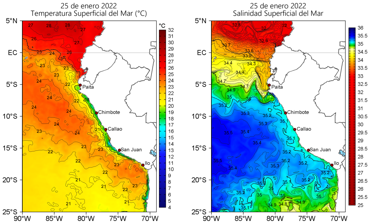
Figura 2. Temperatura superficial del mar (a la izquierda) y Salinidad superficial del mar (a la derecha) para el 25 de enero de 2022. Datos: OSTIA-UKMO-L4-GLOB-v2.0 (UK Met Office, 2012; Donlon et al, 2012) y Hybrid Coordinate Ocean Model v. GOFS 3.1 (HYCOM; Halliwell et al., 1998; 2000; Bleck, 2001), respectivamente.
