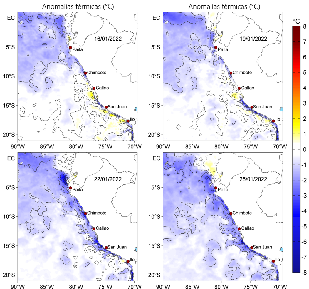
Figura 3. Anomalías de la temperatura superficial del mar (°C) para el 16, 19, 22 y 25 de enero de 2022. Las anomalías se calcularon respecto de la climatología para el periodo 2007-2016. Datos: OSTIA-UKMO-L4-GLOB-v2.0 (UK Met Office, 2012; Donlon et al, 2012).
